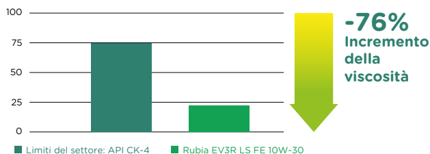
Volvo T13 Test (KV 40 Aumento della viscosità 300-360h)
