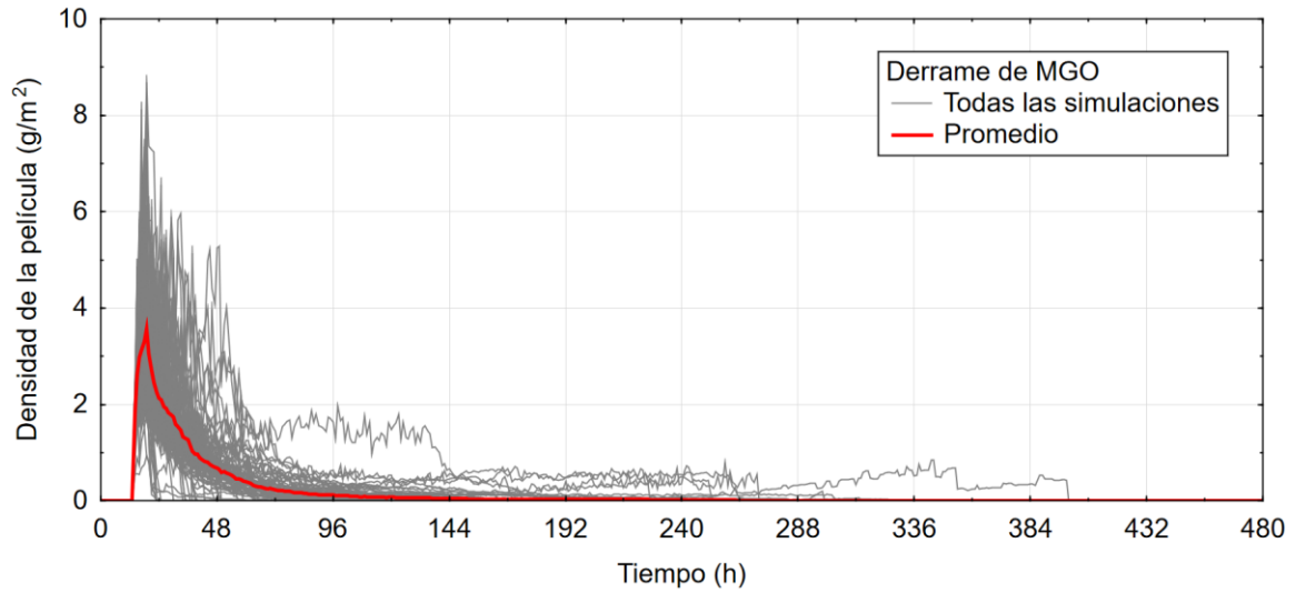
Figura 6.4.5 Resultados de la simulaciones del derrame del MGO Fenix. Densidad de la película del hidrocarburo máxima observada durante las 96 simulaciones realizadas (cobertura temporal de 4 años). Series de tiempo superpuestas de las 96 simulaciones y el valor promedio de cada instante (arriba). Series de tiempo superpuestas de las 96 simulaciones y los valores de referencia asociados a las zonas de alta, moderada y baja exposición (medio). Distribución espacial de las máximas densidades observadas durante las 96 simulaciones.
