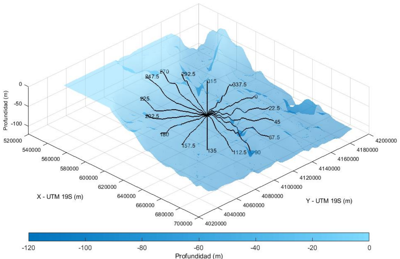
Figura 7.17.1 Batimetría y cortes batimétricos a partir de la fuente en el punto Fenix para todas las direcciones, cada 22.5°. Siendo el N=0°, E=90°, S=180° y O=270°.
