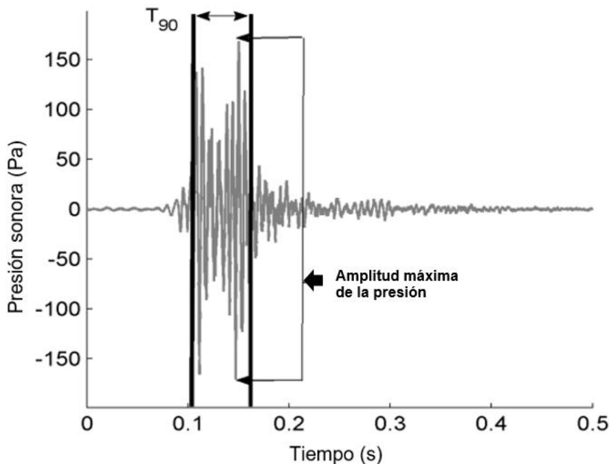
Figura 7.5.1 Forma de onda de presión debida a un solo golpe sobre un pilote. Las líneas verticales en negra indican el inicio y el final de T_{90} . Esta duración incluye al 90% de la energía de la señal (entre el 5% y el 95%). En este caso, el T_{90} es 0.060s (o 60ms, ms: milisegundos), aproximadamente. Gráfico en base a (Leunissen, 2017).
