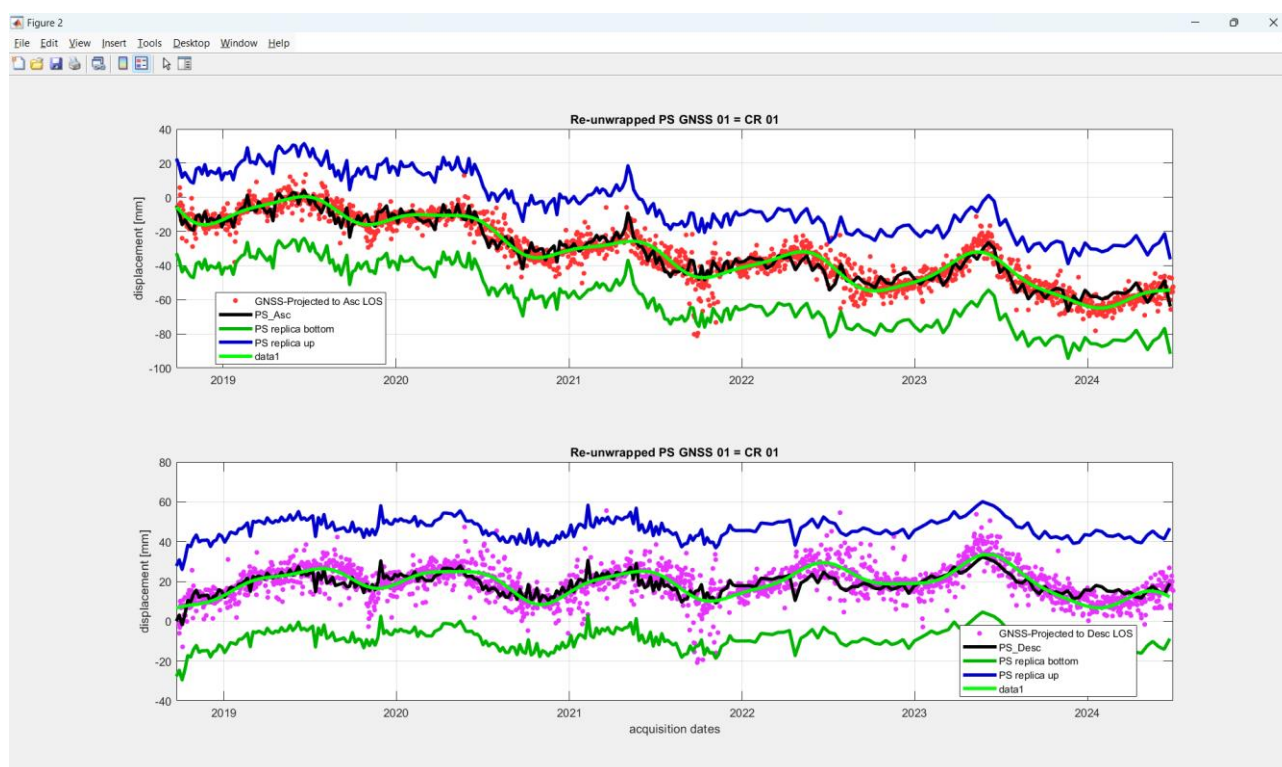
Figura 39: la figura in alto riporta la proiezione delle misure GNSS in corrispondenza del Corner Reflector CR01 (punti rossi) sulla viste SAR ascending mentre la figura in basso riporta la proiezione delle misure GNSS sulla vista SAR descending (punti viola) e raffronto con le misure SAR rappresentate dalla linea nera (le linee blu e verdi rappresentano le due repliche delle misure SAR di una quantità pari a \pm \lambda/2 ). Si nota un ottimo accordo a livello qualitativo.
