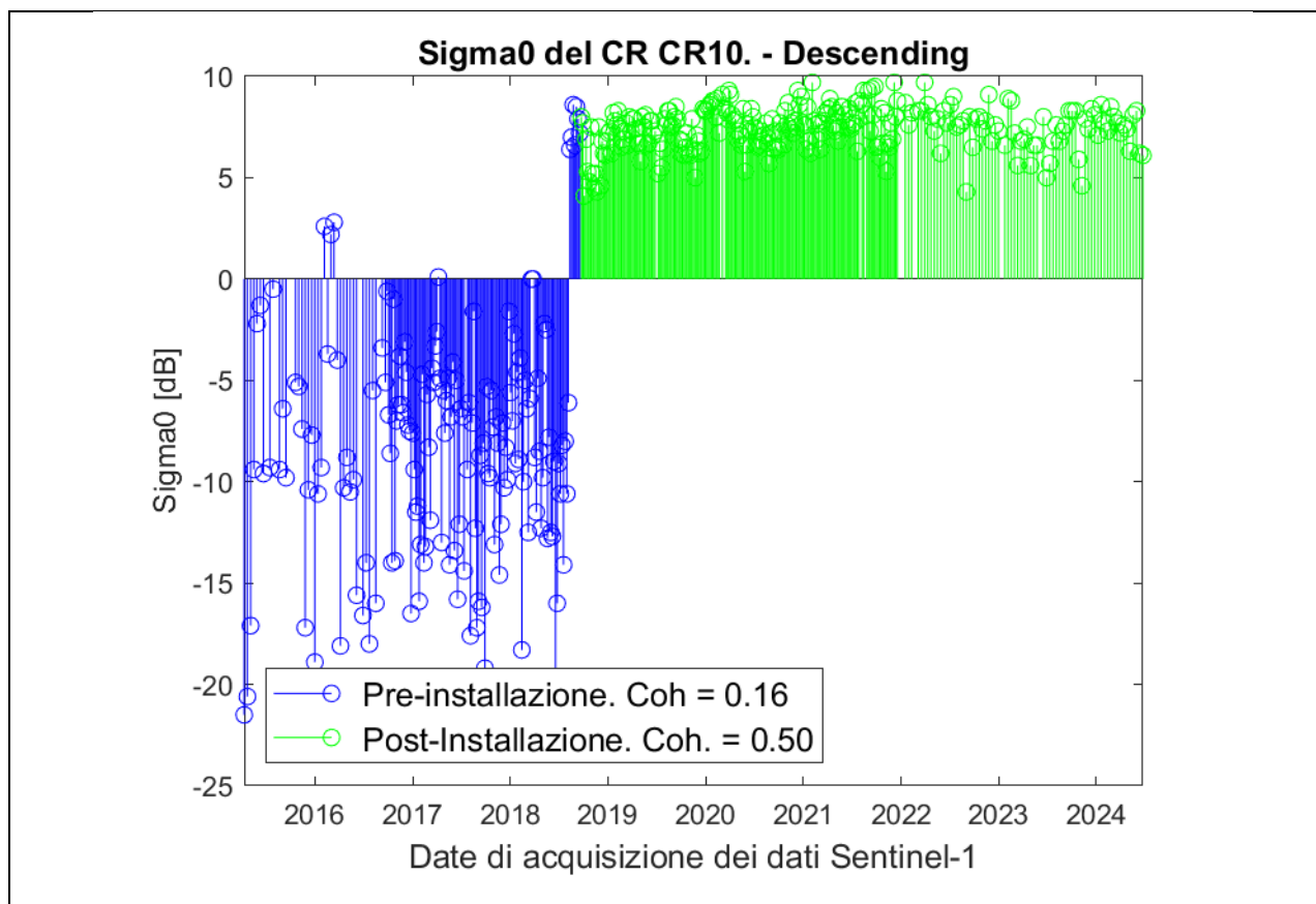
Fig. 0.40: Analisi radiometrica della serie temporale (modalità descending) in corrispondenza del corner reflector CR10. In blu sono indicate le misure pre-installazione. In verde sono indicate le misure post-installazione.
