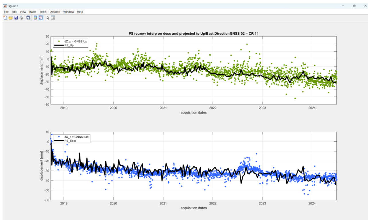
Figura 43: la figura in alto riporta la proiezione delle misure SAR in corrispondenza del Corner Reflector CR11 in direzione verticale (linea nera) unitamente alle misure di spostamento verticale GNSS (punti verdi) mentre la figura in basso riporta la proiezione delle misure SAR in direzione est (linea nera) unitamente alle misure GNSS nella stessa direzione (punti blu). Si nota un ottimo accordo a livello qualitativo.
