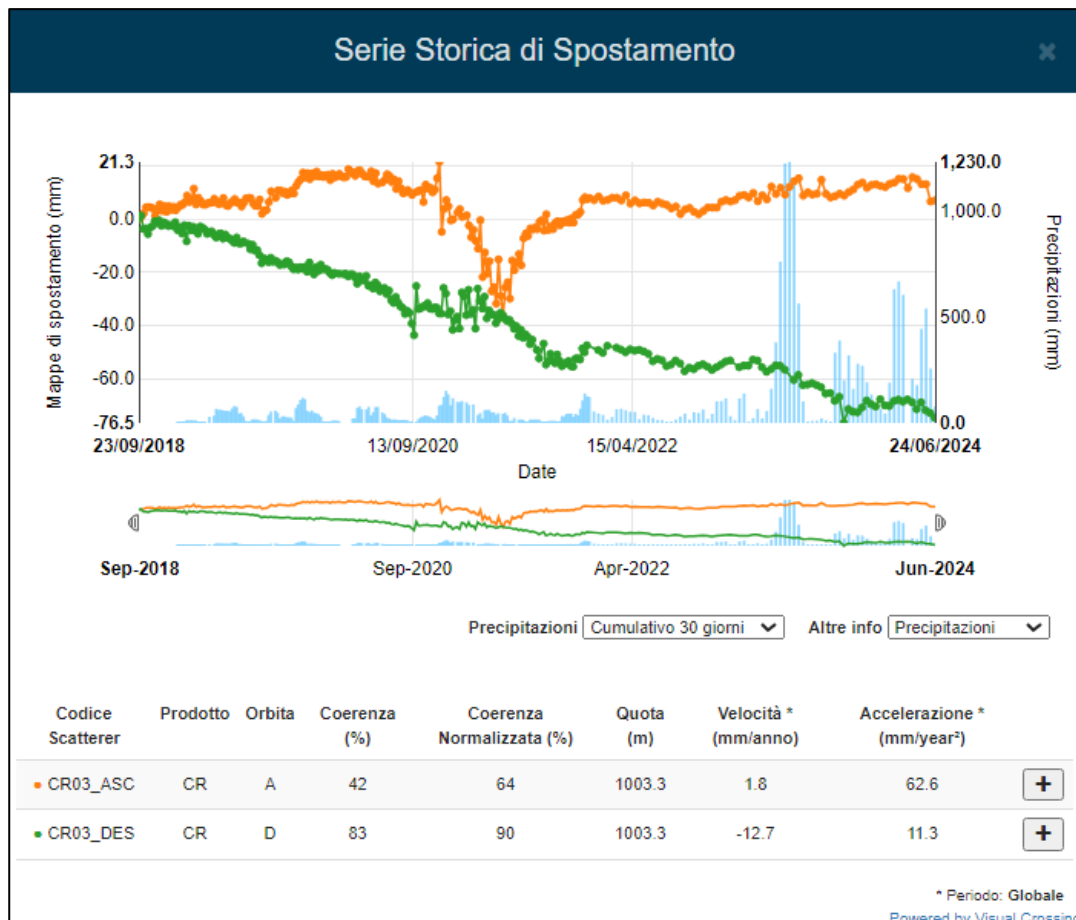
Figura 25: serie temporale di spostamento relativa al periodo settembre 2018 – Giugno 2024 misurata in corrispondenza del Corner Reflector CR03. La serie temporale di spostamento in verde è relativa all'orbita Descending mentre quella arancione rappresenta la serie temporale relativa all'orbita Ascending.
