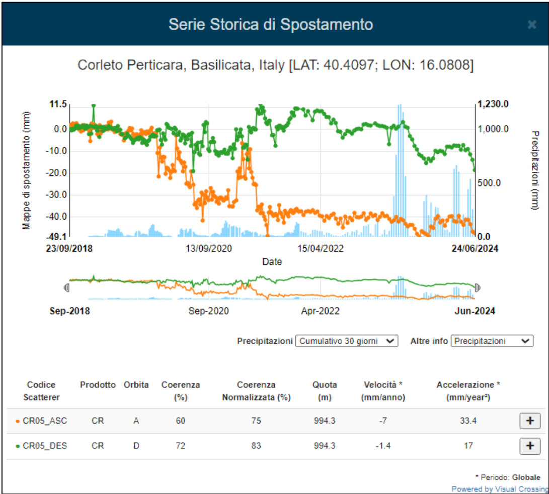
Figura 13: serie temporale di spostamento relativa al periodo settembre 2018 – Giugno 2024 misurata in corrispondenza del Corner Reflector CR05. La serie temporale di spostamento in arancione è relativa all'orbita Ascending mentre quella verde rappresenta la serie temporale relativa all'orbita Descending.
