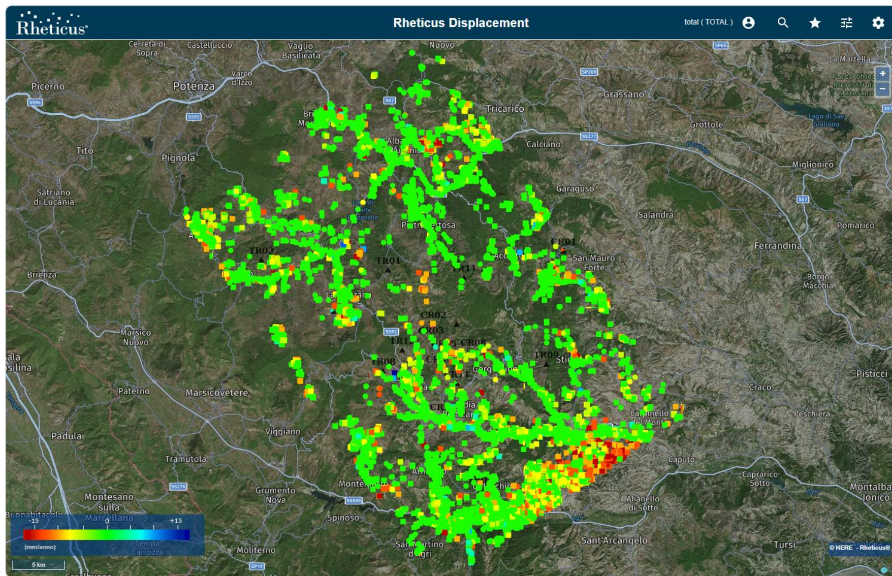
Figura 3: Mappa velocità media annua (mm/anno) lungo la LOS sul periodo esteso a Giugno 2024 ottenuta dal processamento del dataset Sentinel-1 in orbita ascending.
