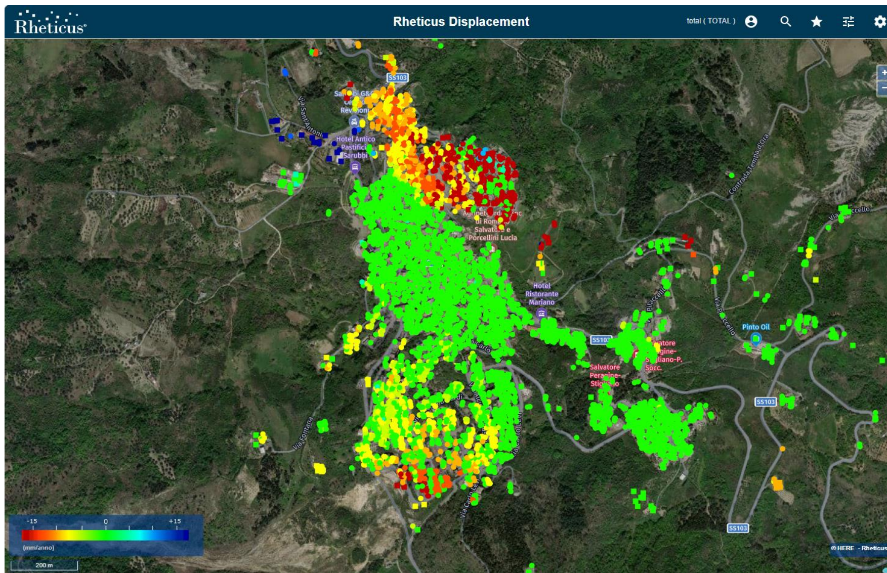
Figura 9: La mappa di velocità media (mm/anno) PS/DS sul centro abitato di Stigliano calcolata sul periodo esteso a Giugno 2024 non mostra variazioni significative rispetto al rapporto precedente [RD16].
