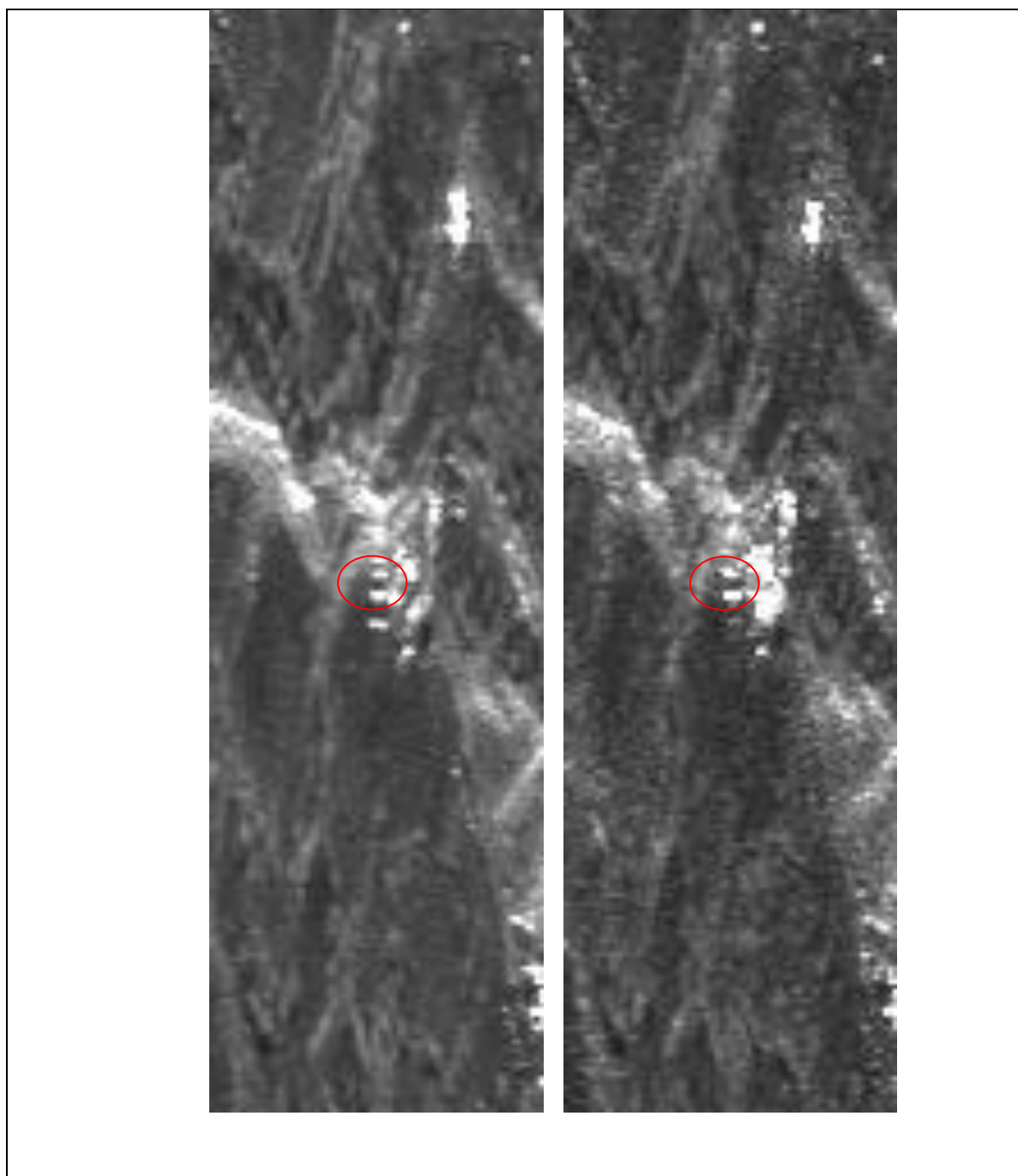
Fig. 0.31: Immagini di intensità in modalità descending centrate sul corner reflector CR08. A sinistra: immagine pre-installazione. A destra: immagine post-installazione. Il cerchio di colore rosso indica la posizione del corner reflector.
