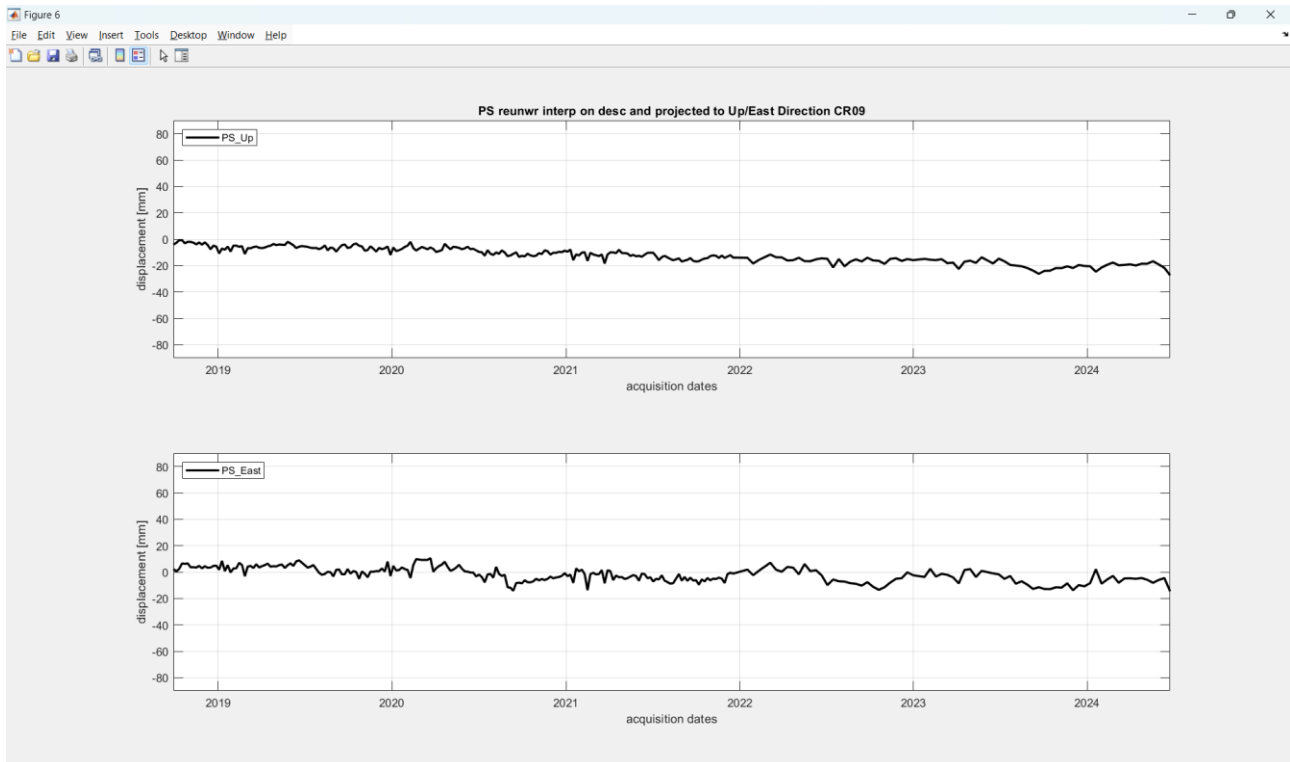
Figura 29: il grafico in alto rappresenta la serie temporale di spostamento in direzione Verticale (PS_Up) mentre il grafico in basso rappresenta la serie temporale di spostamento in direzione est (PS_Est).
