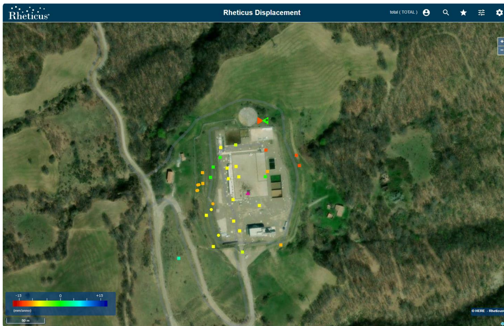
Figura 18: Pozzo TE-1 (indicato dal triangolo fucsia) caratterizzato da una buona copertura di PS e dai quali nel periodo esteso a Giugno 2024, non si evincono variazioni significative di velocità media rispetto al precedente rapporto [RD16].
