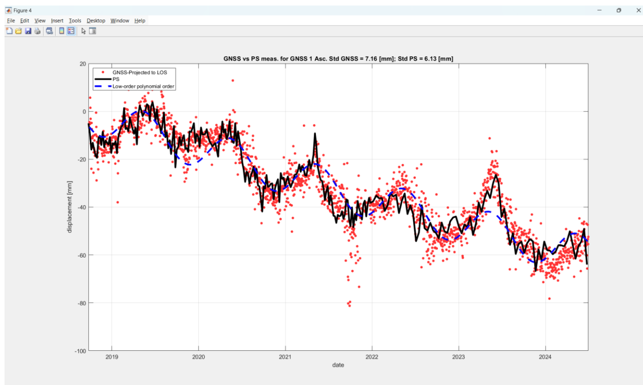
Figura 45: la figura rappresenta il confronto quantitativo effettuato in geometria SAR Ascending tra le misure GNSS (punti rossi) e SAR (linea nera) in corrispondenza del CR01. La linea blu tratteggiata rappresenta il fit polinomiale stimato sui dati GNSS. Il trend delle serie temporali GNSS e SAR e le relative deviazioni standard confermano un ottimo accordo anche a livello quantitativo.
