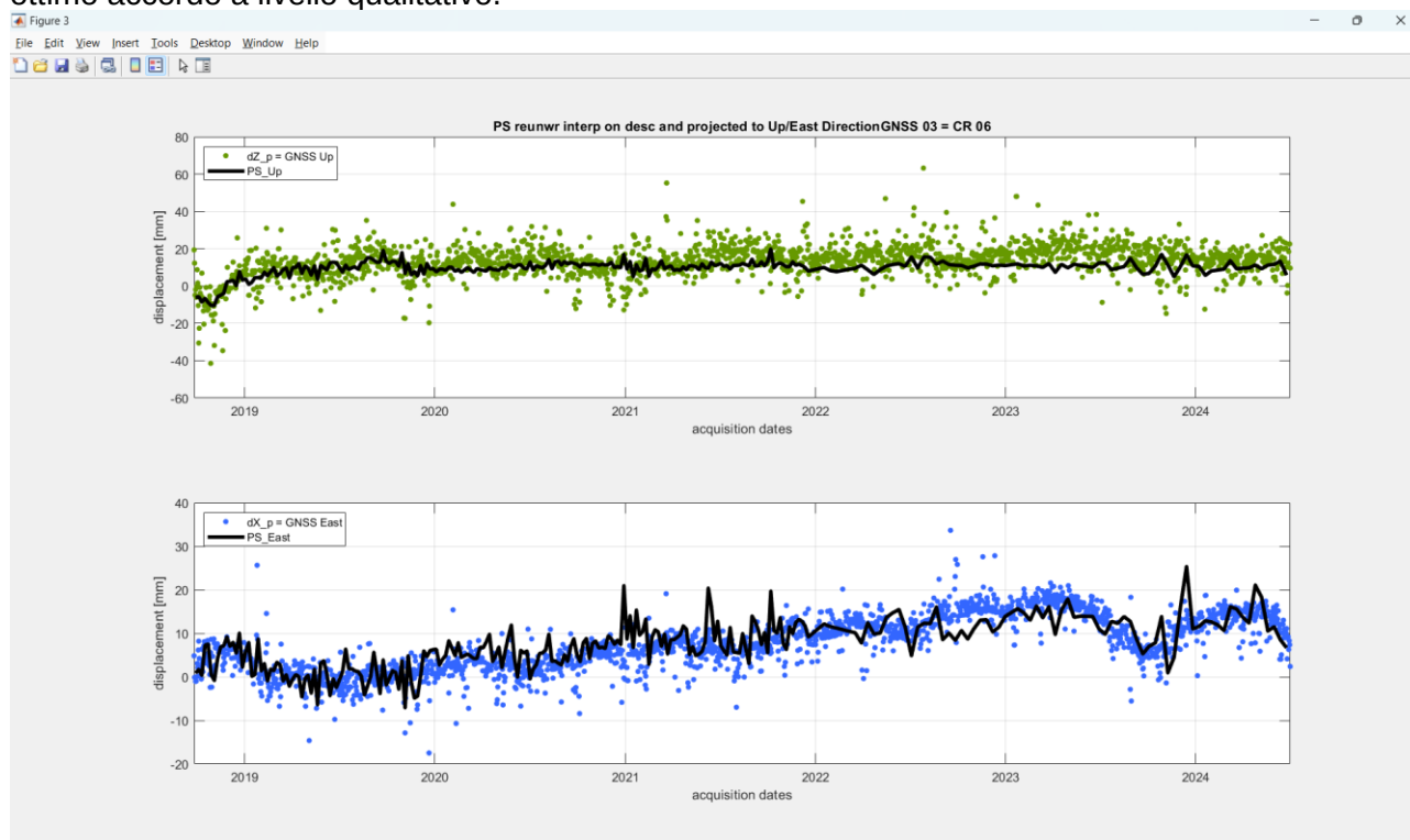
Figura 44: la figura in alto riporta la proiezione delle misure SAR in corrispondenza del Corner Reflector CR06 in direzione verticale (linea nera) unitamente alle misure di spostamento verticale GNSS (punti verdi) mentre la figura in basso riporta la proiezione delle misure SAR in direzione est (linea nera) unitamente alle misure GNSS nella stessa direzione (punti blu). Si nota un ottimo accordo a livello qualitativo.
