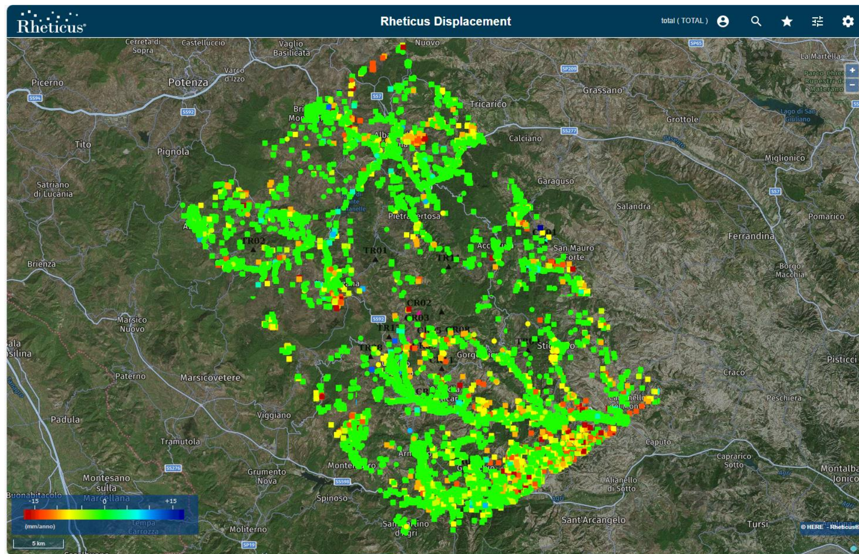
Figura 4: Mappa velocità media annua (mm/anno) lungo la LOS sul periodo esteso a Giugno 2024 ottenuta dal processamento del dataset Sentinel-1 in orbita descending.
