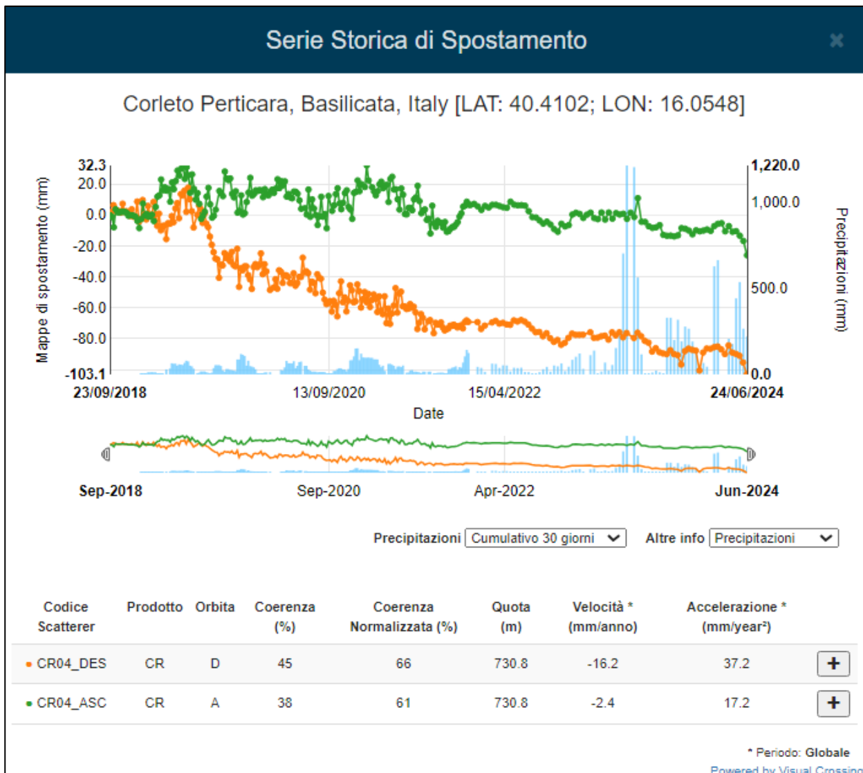
Figura 22: serie temporale di spostamento relativa al periodo settembre 2018 – Giugno 2024 misurata in corrispondenza del Corner Reflector CR04. La serie temporale di spostamento in verde è relativa all'orbita Ascending mentre quella arancione rappresenta la serie temporale relativa all'orbita Descending.
