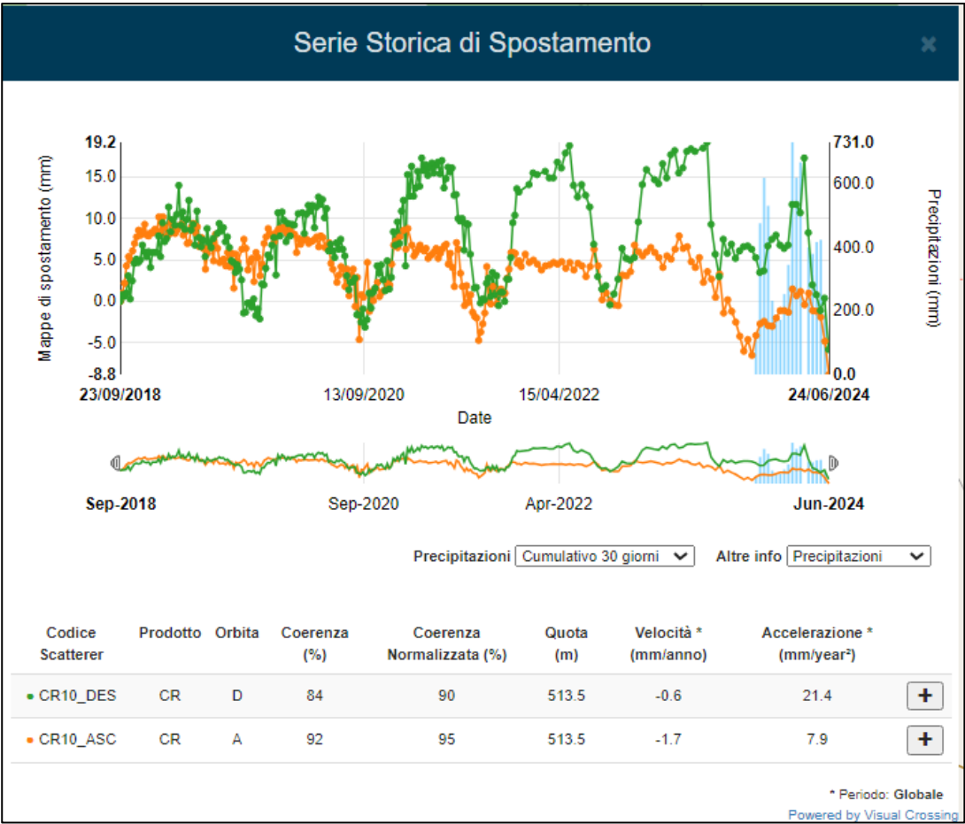
Figura 31: serie temporale di spostamento relativa al periodo settembre 2018 – Giugno 2024 misurata in corrispondenza del Corner Reflector CR10. La serie temporale di spostamento in verde è relativa all’orbita Descending mentre quella arancione rappresenta la serie temporale relativa all’orbita Ascending.
