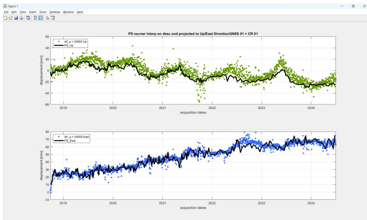
Figura 42: la figura in alto riporta la proiezione delle misure SAR in corrispondenza del Corner Reflector CR01 in direzione verticale (linea nera) unitamente alle misure di spostamento verticale GNSS (punti verdi) mentre la figura in basso riporta la proiezione delle misure SAR in direzione est (linea nera) unitamente alle misure GNSS nella stessa direzione (punti blu). Si nota un buon accordo a livello qualitativo.
