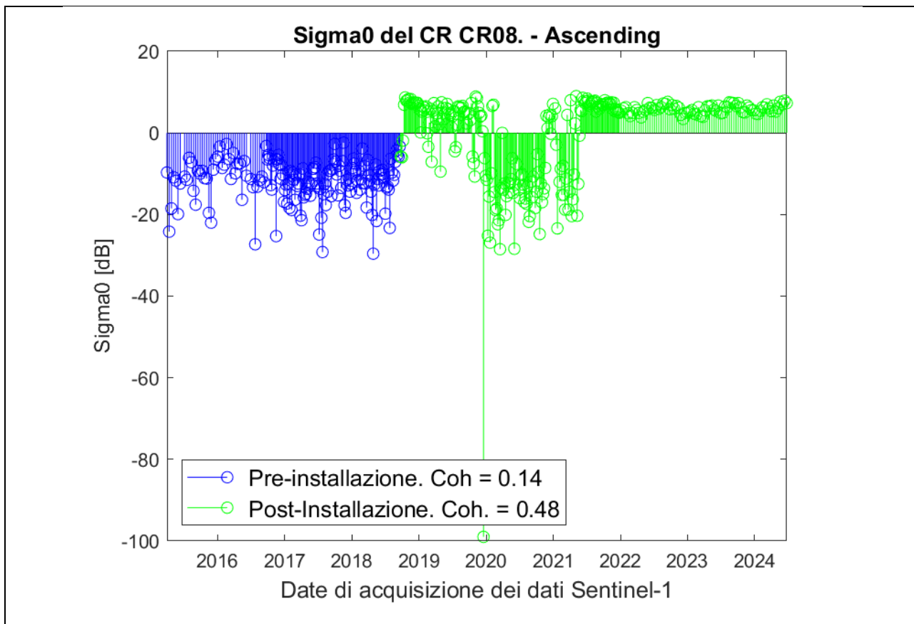
Fig. 0.30: Analisi radiometrica della serie temporale (modalità ascending) in corrispondenza del corner reflector CR08. In blu sono indicate le misure pre-installazione. In verde sono indicate le misure post-installazione.
