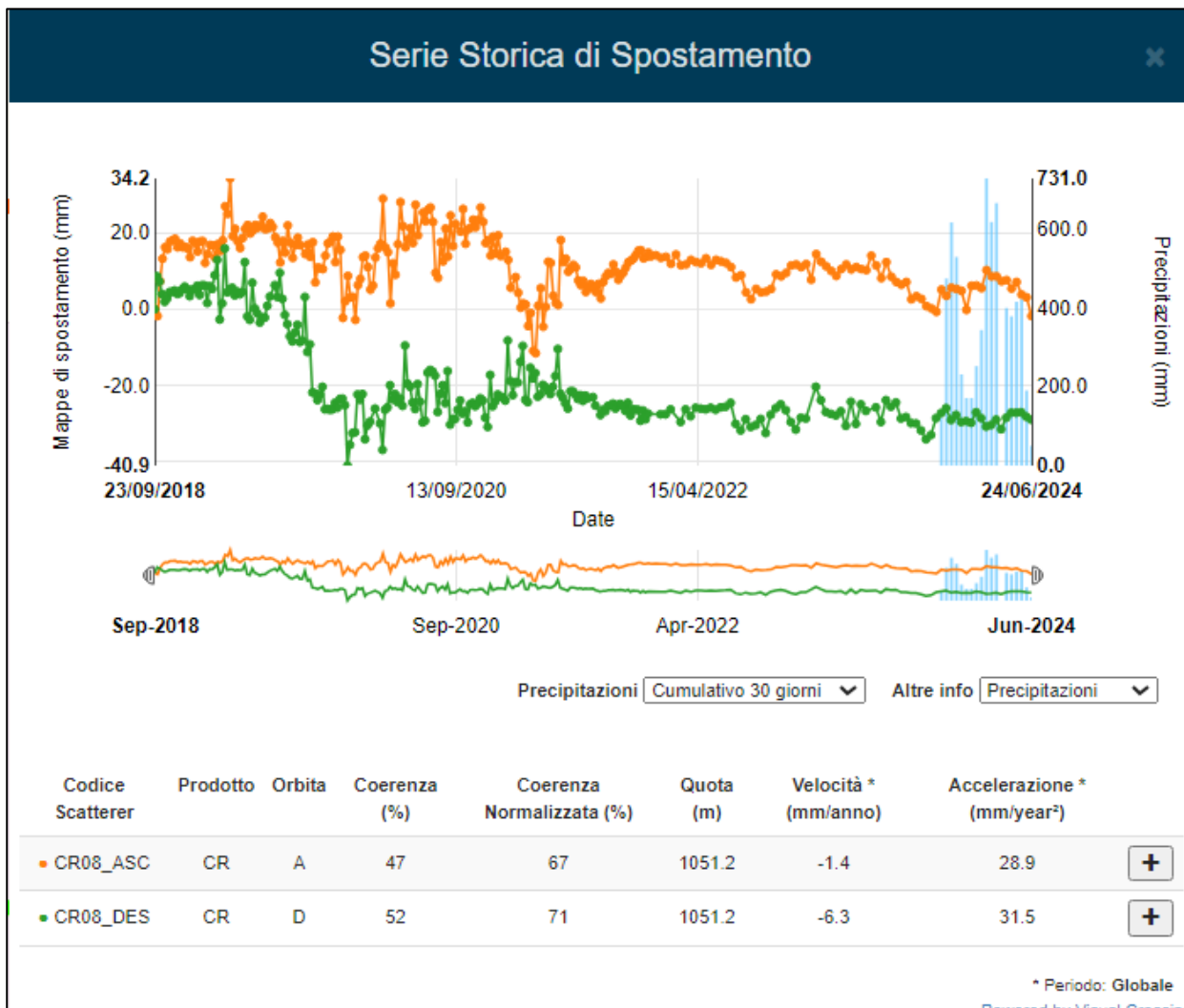
Figura 16: serie temporale di spostamento relativa al periodo settembre 2018 – Giugno 2024 misurata in corrispondenza del Corner Reflector CR08. La serie temporale di spostamento in arancione è relativa all'orbita Ascending mentre quella verde rappresenta la serie temporale relativa all'orbita Descending.
