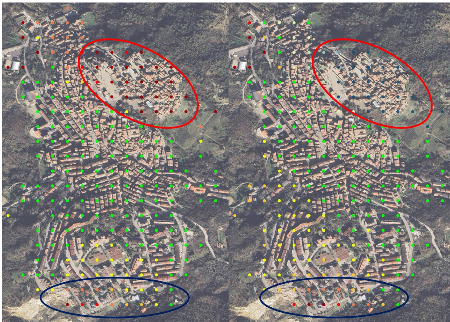
Figura 11: La mappa delle componenti di velocità media Est(+) – Ovest(-) (immagine di destra) e Verticale (immagine di sinistra) sul centro abitato di Stigliano calcolata sul periodo esteso a Giugno 2024 è in linea con quanto misurato nel rapporto precedente [RD16]. Sulla zona nord (evidenziata dal poligono rosso nelle immagini) si evince una velocità media in direzione Est pari a circa 19.7 mm/anno e una componente di abbassamento verticale medio pari a -15.0 mm/anno mentre la zona sud-ovest (evidenziata dal poligono blu nelle immagini) presenta uno spostamento medio in direzione Ovest pari a -5.5 mm/anno fino ad un massimo di -11.5 mm/anno e una componente di abbassamento verticale media pari a -5.0 mm/anno fino ad un massimo di -12.0 mm/anno.
