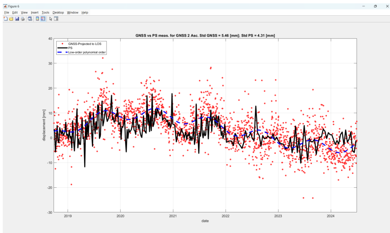
Figura 47: la figura rappresenta il confronto quantitativo effettuato in geometria SAR Ascending tra le misure GNSS (punti rossi) e SAR (linea nera) in corrispondenza del CR11. La linea blu tratteggiata rappresenta il fit polinomiale stimato sui dati GNSS. Il trend delle serie temporali GNSS e SAR e le relative deviazioni standard confermano un ottimo accordo anche a livello quantitativo.
