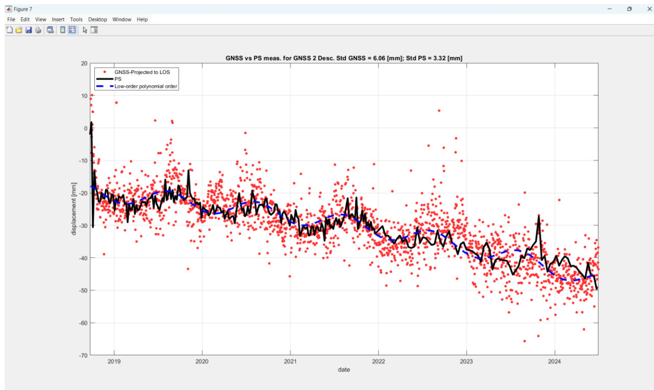
Figura 48: la figura rappresenta il confronto quantitativo effettuato in geometria SAR Descending tra le misure GNSS (punti rossi) e SAR (linea nera) in corrispondenza del CR11. La linea blu tratteggiata rappresenta il fit polinomiale stimato sui dati GNSS. Il trend delle serie temporali GNSS e SAR e le relative deviazioni standard confermano un ottimo accordo anche a livello quantitativo.
