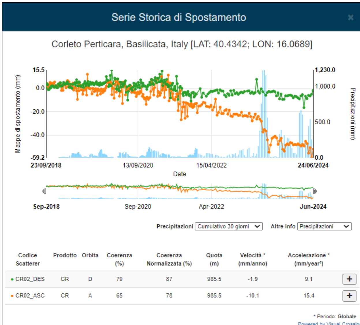
Figura 19: serie temporale di spostamento relativa al periodo settembre 2018 – Giugno 2024 misurata in corrispondenza del Corner Reflector CR02. La serie temporale di spostamento in verde è relativa all'orbita Descending mentre quella arancione rappresenta la serie temporale relativa all'orbita Ascending.
