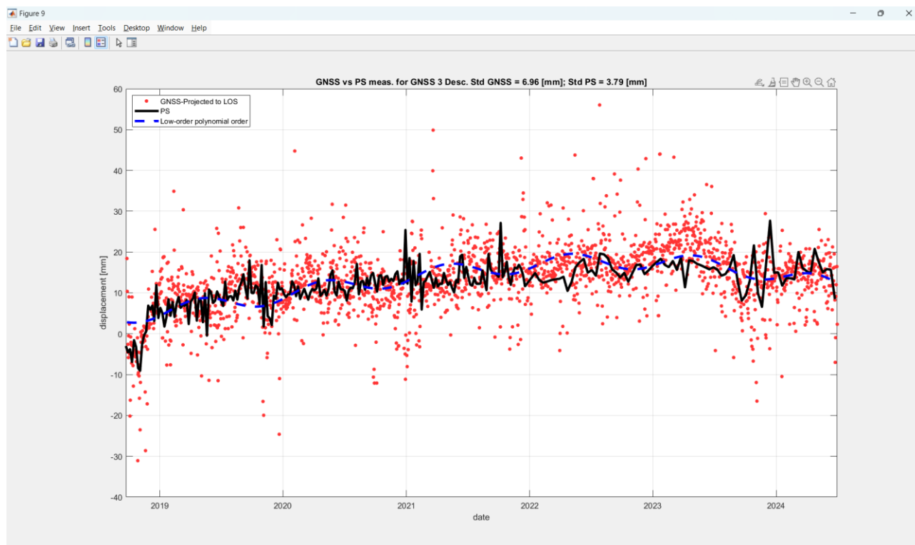
Figura 50: la figura rappresenta il confronto quantitativo effettuato in geometria SAR Descending tra le misure GNSS (punti rossi) e SAR (linea nera) in corrispondenza del CR06. La linea blu tratteggiata rappresenta il fit polinomiale stimato sui dati GNSS. Il trend delle serie temporali GNSS e SAR e le relative deviazioni standard confermano un ottimo accordo anche a livello quantitativo.
