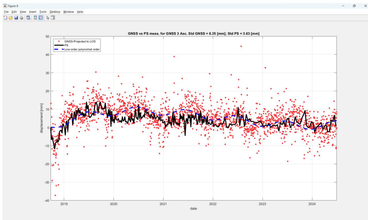
Figura 49: la figura rappresenta il confronto quantitativo effettuato in geometria SAR Ascending tra le misure GNSS (punti rossi) e SAR (linea nera) in corrispondenza del CR06. La linea blu tratteggiata rappresenta il fit polinomiale stimato sui dati GNSS. Il trend delle serie temporali GNSS e SAR e le relative deviazioni standard confermano un ottimo accordo anche a livello quantitativo.
