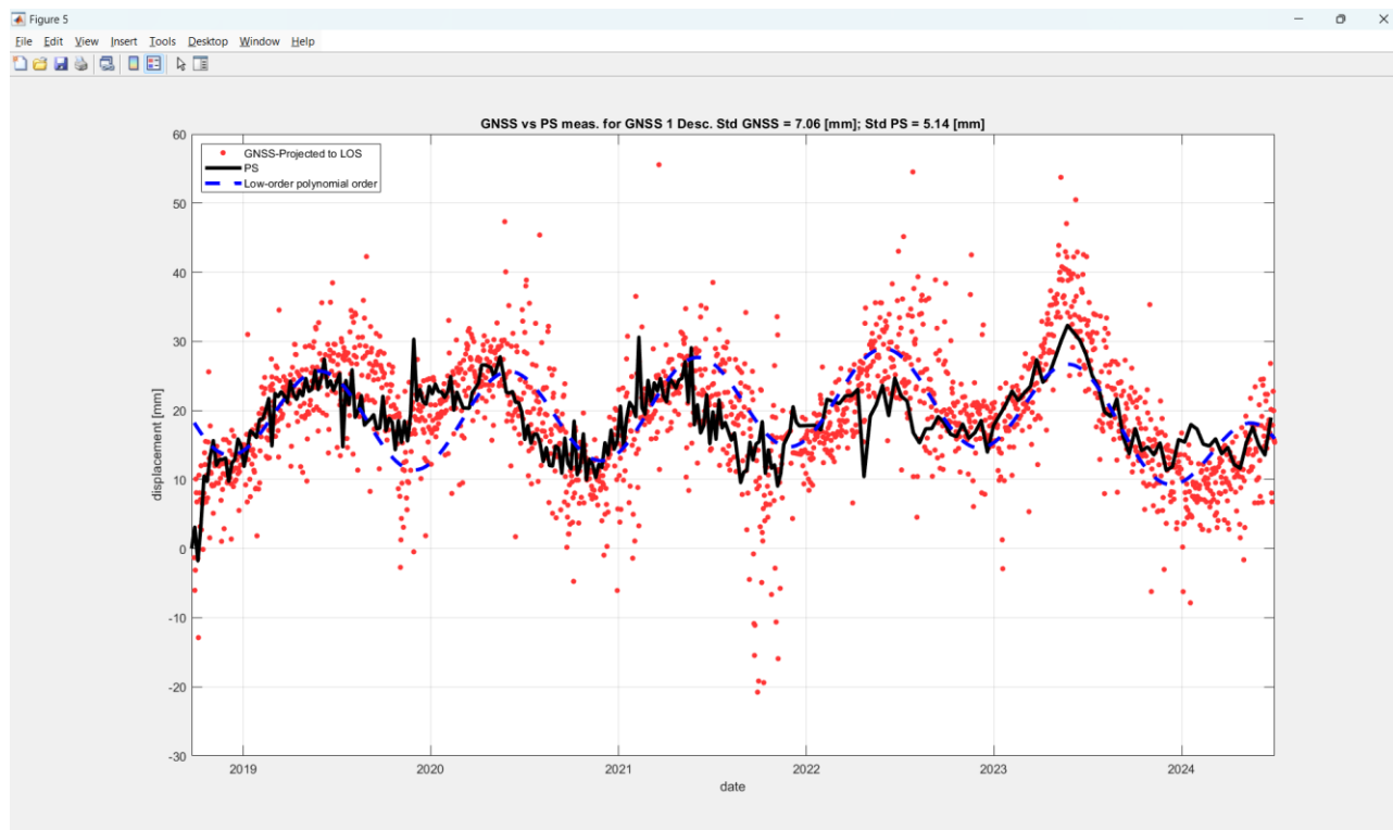
Figura 46: la figura rappresenta il confronto quantitativo effettuato in geometria SAR Descending tra le misure GNSS (punti rossi) e SAR (linea nera) in corrispondenza del CR01. La linea blu tratteggiata rappresenta il fit polinomiale stimato sui dati GNSS. Il trend delle serie temporali GNSS e SAR e le relative deviazioni standard confermano un ottimo accordo anche a livello quantitativo.
