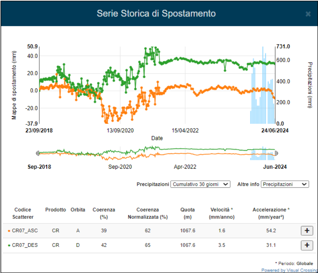
Figura 34: serie temporale di spostamento relativa al periodo settembre 2018 – Giugno 2024 misurata in corrispondenza del Corner Reflector CR07. La serie temporale di spostamento in verde è relativa all'orbita Descending mentre quella arancione rappresenta la serie temporale relativa all'orbita Ascending.
