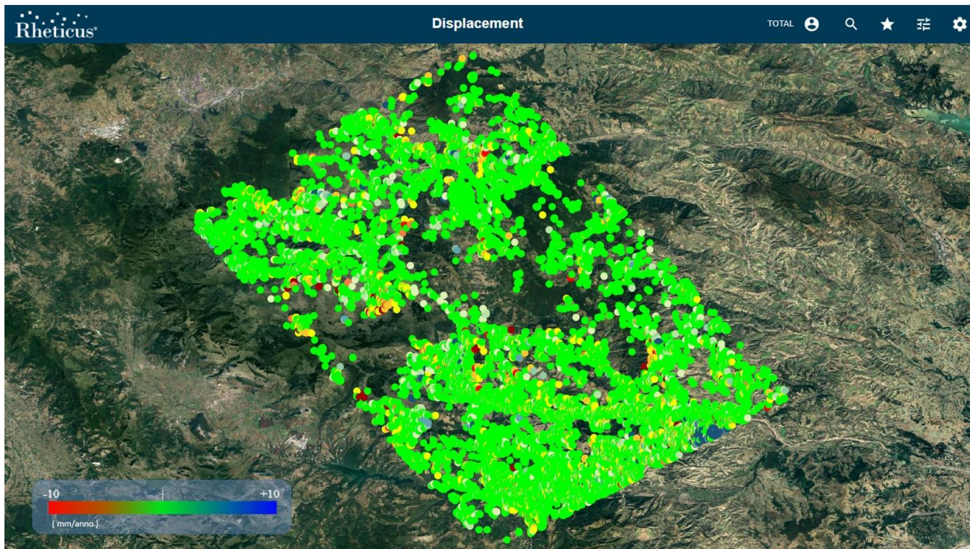
Figura 6: Mappa velocità media annua (mm/anno) in direzione Est(+) - Ovest(-) sul periodo esteso a Giugno 2024 ottenuta dalla combinazione delle immagini Ascending e Descending acquisite dal satellite Sentinel-1.
