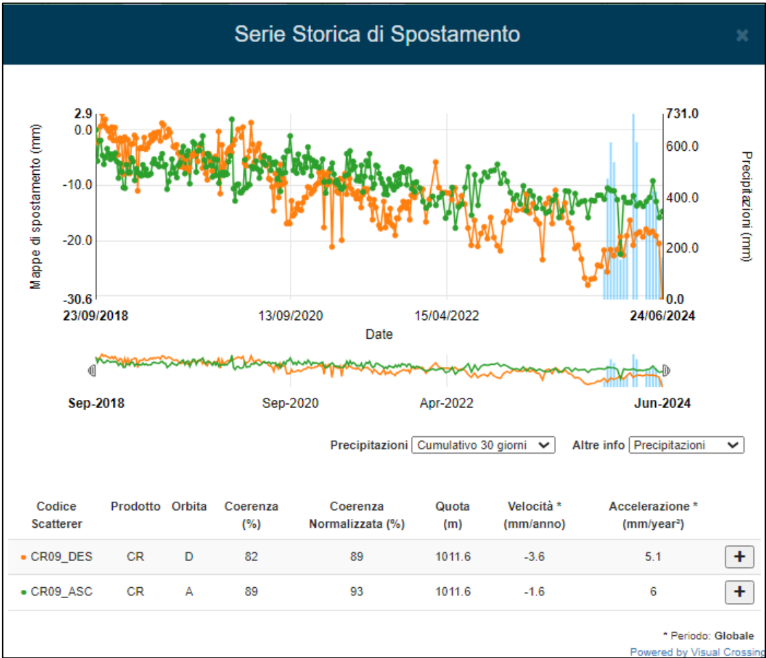
Figura 28: serie temporale di spostamento relativa al periodo settembre 2018 – Giugno 2024 misurata in corrispondenza del Corner Reflector CR09. La serie temporale di spostamento in verde è relativa all’orbita Ascending mentre quella arancione rappresenta la serie temporale relativa all’orbita Descending.
