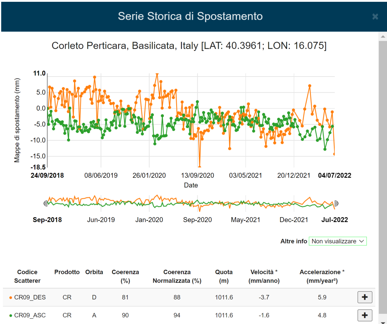
Figura 28: serie temporale di spostamento relativa al periodo settembre 2018 – Giugno 2022 misurata in corrispondenza del Corner Reflector CR09. La serie temporale di spostamento in verde è relativa all’orbita Ascending mentre quella arancione rappresenta la serie temporale relativa all’orbita Descending.
