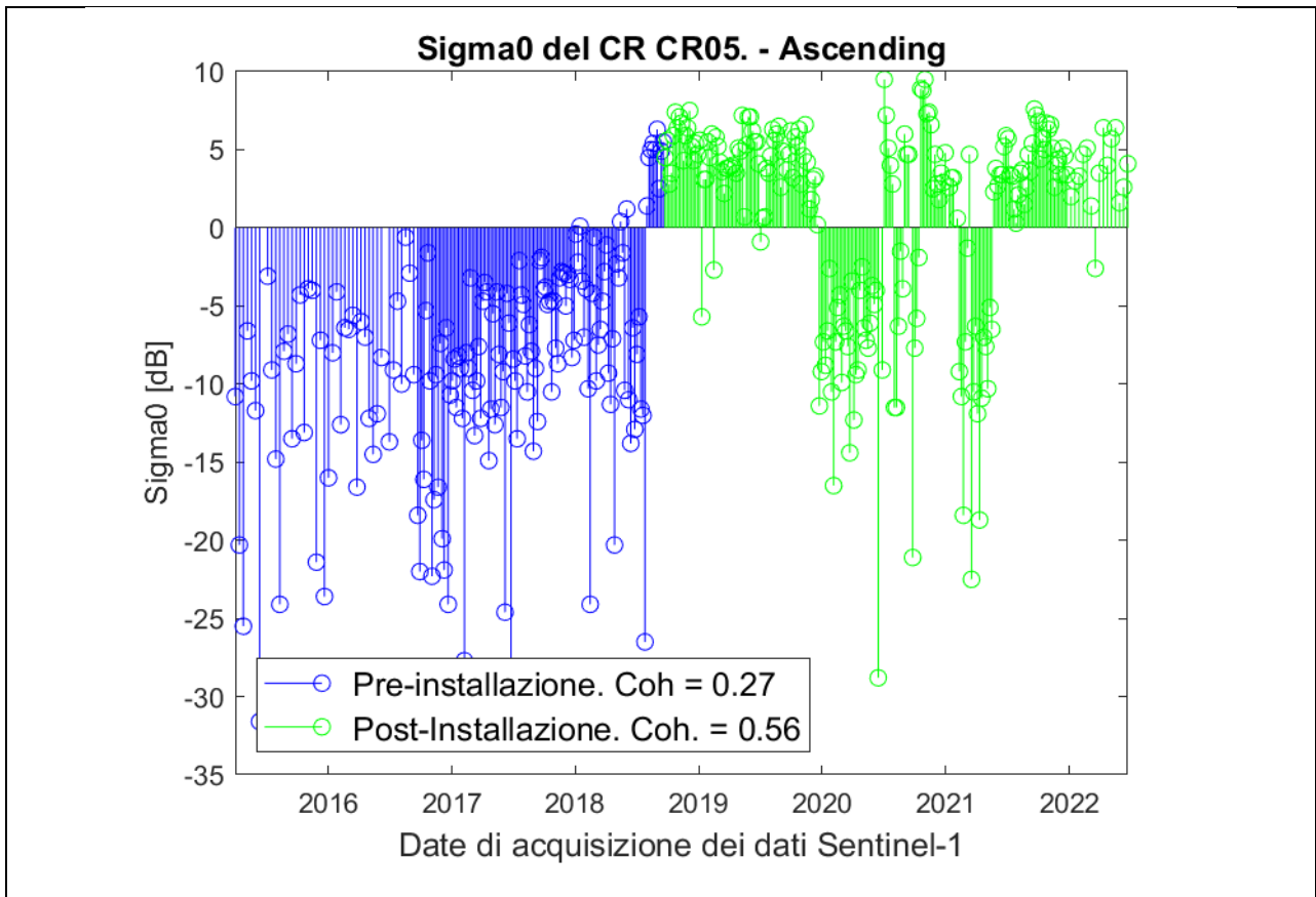
Fig. 0.18: Analisi radiometrica della serie temporale (modalità ascending) in corrispondenza del corner reflector CR05. In blu sono indicate le misure pre-installazione. In verde sono indicate le misure post-installazione.
