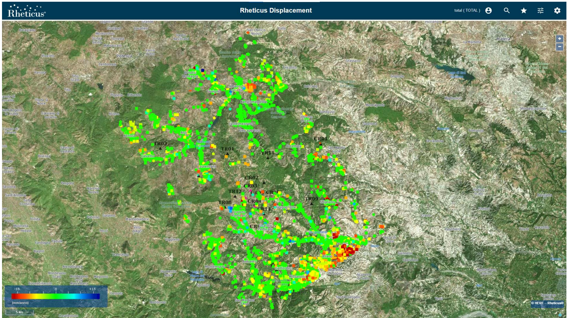
Figura 3: Mappa velocità media annua (mm/anno) lungo la LOS sul periodo esteso a Giugno 2022 ottenuta dal processamento del dataset Sentinel-1 in orbita ascending.
