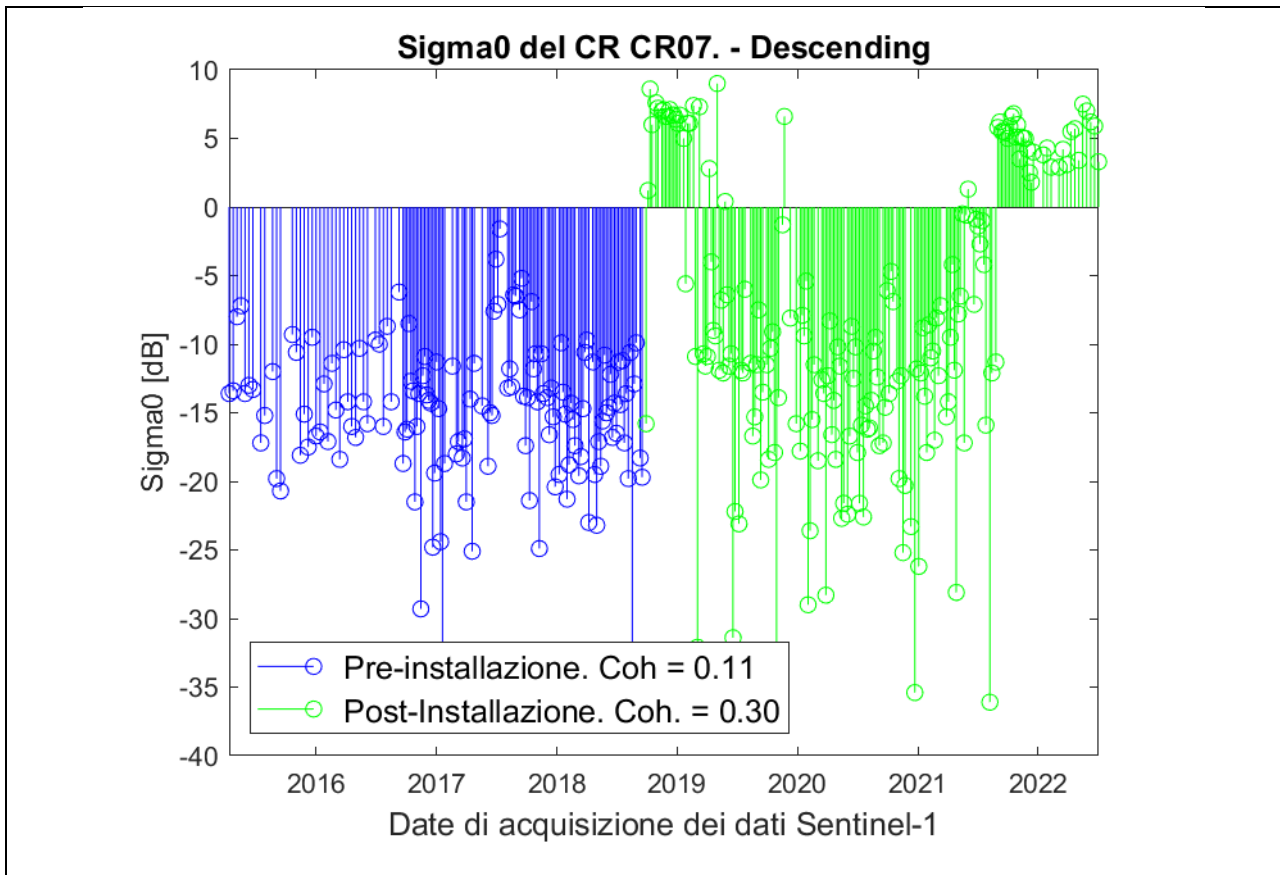
Fig. 0.28: Analisi radiometrica della serie temporale (modalità descending) in corrispondenza del corner reflector CR07. In blu sono indicate le misure pre-installazione. In verde sono indicate le misure post-installazione. Una corretta installazione del corner dovrebbe fare apprezzare nella fase di post-installazione un segnale con maggiore intensità. Nel caso in questione, le misure post-installazione risultano disturbate e con valori di sigma0 molto inferiori ai valori attesi.
