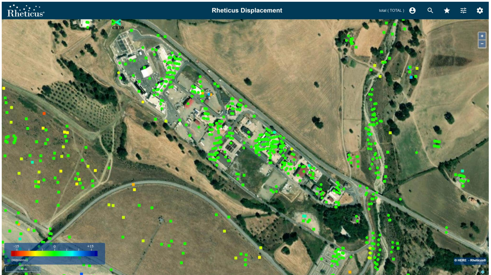
Figura 30: LPG Center caratterizzato da una buona copertura di PS e dai quali nel periodo esteso a Giugno 2022, non si evincono variazioni significative di velocità media rispetto al precedente rapporto [RD12].
