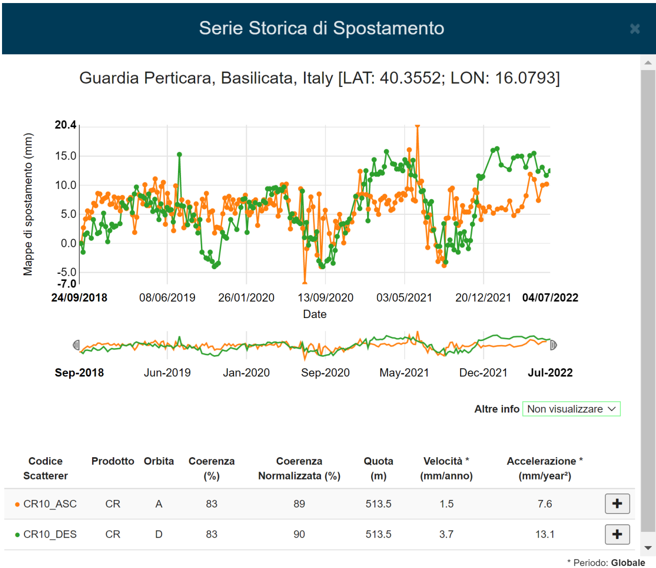
Figura 31: serie temporale di spostamento relativa al periodo settembre 2018 – Giugno 2022 misurata in corrispondenza del Corner Reflector CR10. La serie temporale di spostamento in verde è relativa all'orbita Descending mentre quella arancione rappresenta la serie temporale relativa all'orbita Ascending.
