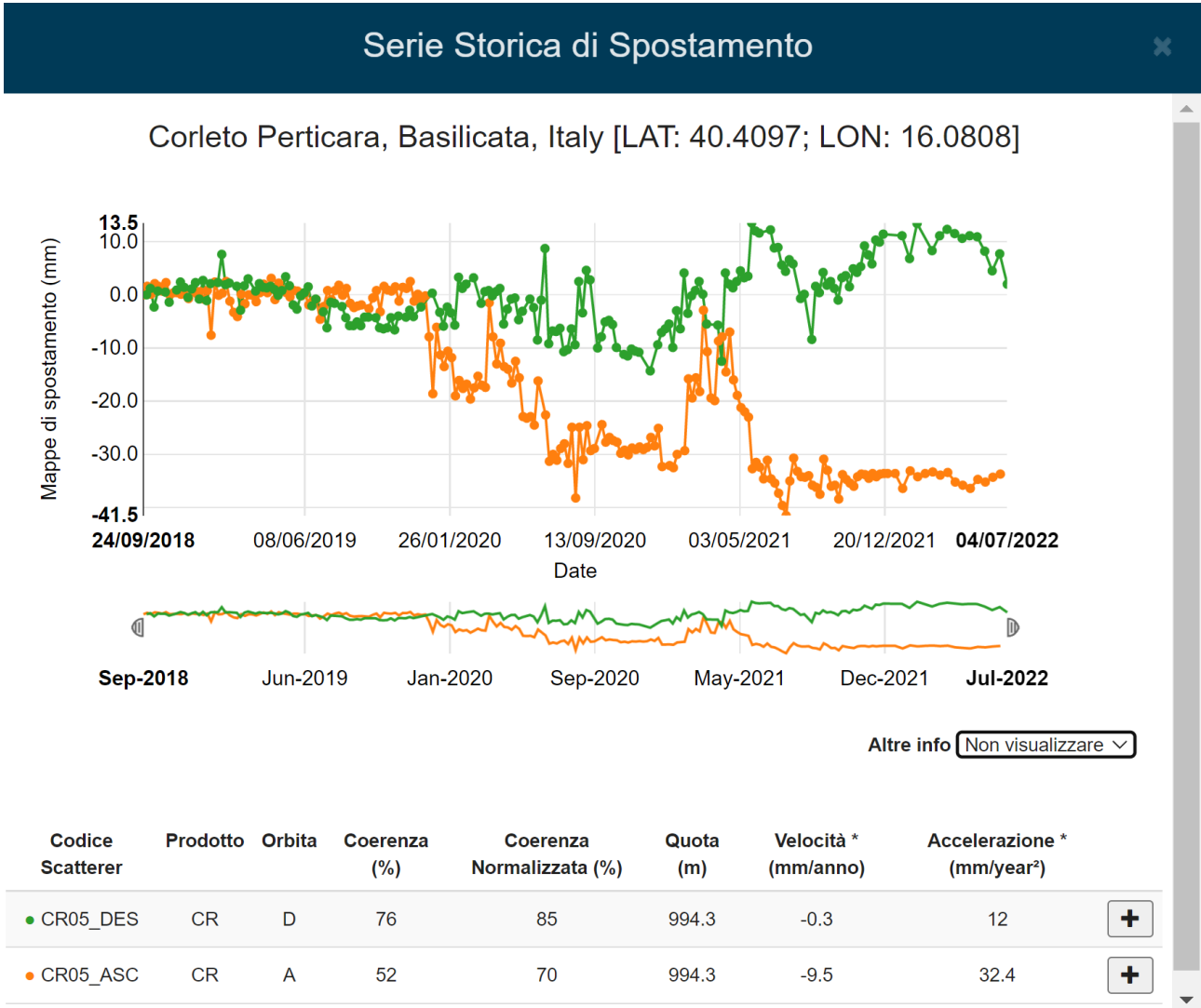
Figura 13: serie temporale di spostamento relativa al periodo settembre 2018 – Giugno 2022 misurata in corrispondenza del Corner Reflector CR05. La serie temporale di spostamento in arancione è relativa all’orbita Ascending mentre quella verde rappresenta la serie temporale relativa all’orbita Descending.
