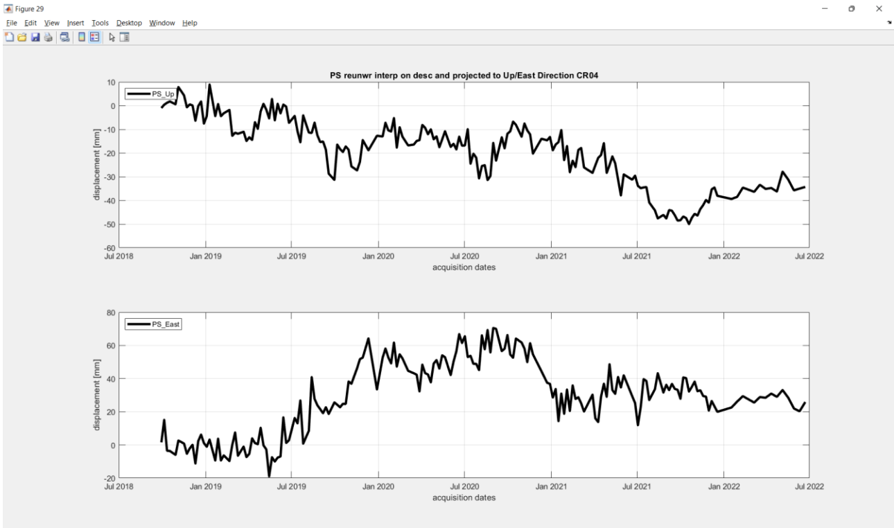
Figura 23: il grafico in alto rappresenta la serie temporale di spostamento in direzione Verticale (PS_Up) mentre il grafico in basso rappresenta la serie temporale di spostamento in direzione est (PS_Est).
