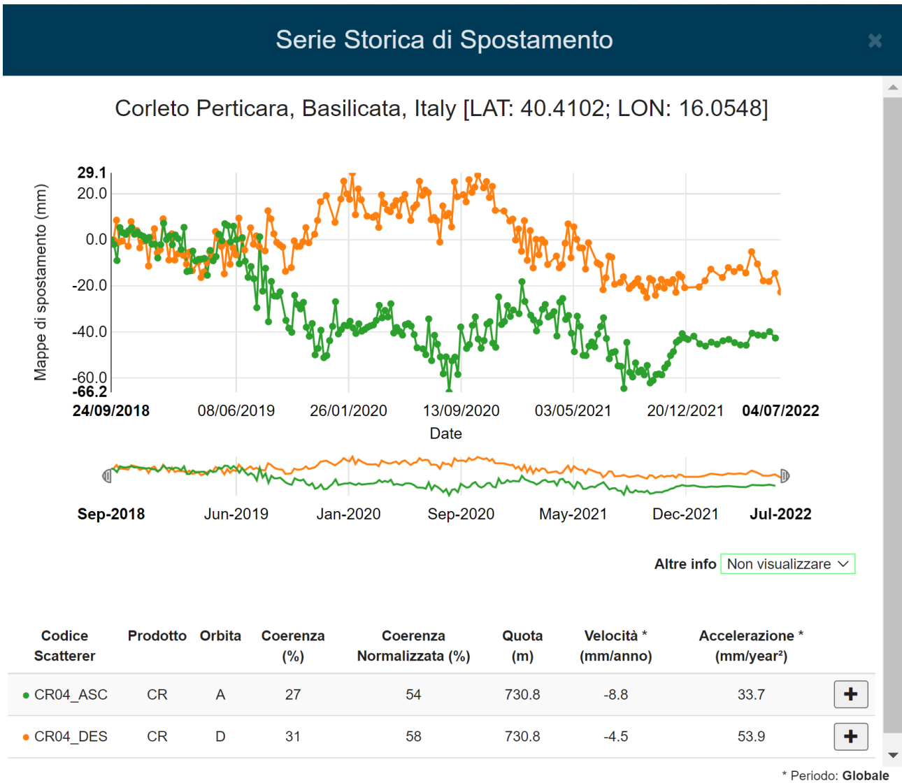
Figura 22: serie temporale di spostamento relativa al periodo settembre 2018 – Giugno 2022 misurata in corrispondenza del Corner Reflector CR04. La serie temporale di spostamento in verde è relativa all’orbita Ascending mentre quella arancione rappresenta la serie temporale relativa all’orbita Descending.
