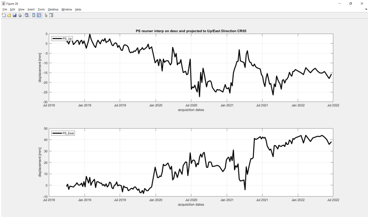
Figura 14: il grafico in alto rappresenta la serie temporale di spostamento in direzione Verticale (PS_Up) mentre il grafico in basso rappresenta la serie temporale di spostamento in direzione est (PS_Est).
