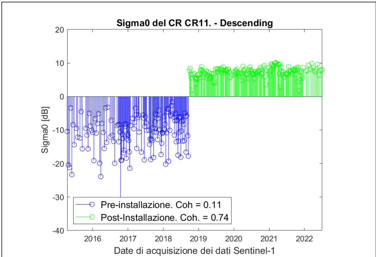
Fig. 0.44: Analisi radiometrica della serie temporale (modalità descending) in corrispondenza del corner reflector CR11. In blu sono indicate le misure pre-installazione. In verde sono indicate le misure post-installazione.
