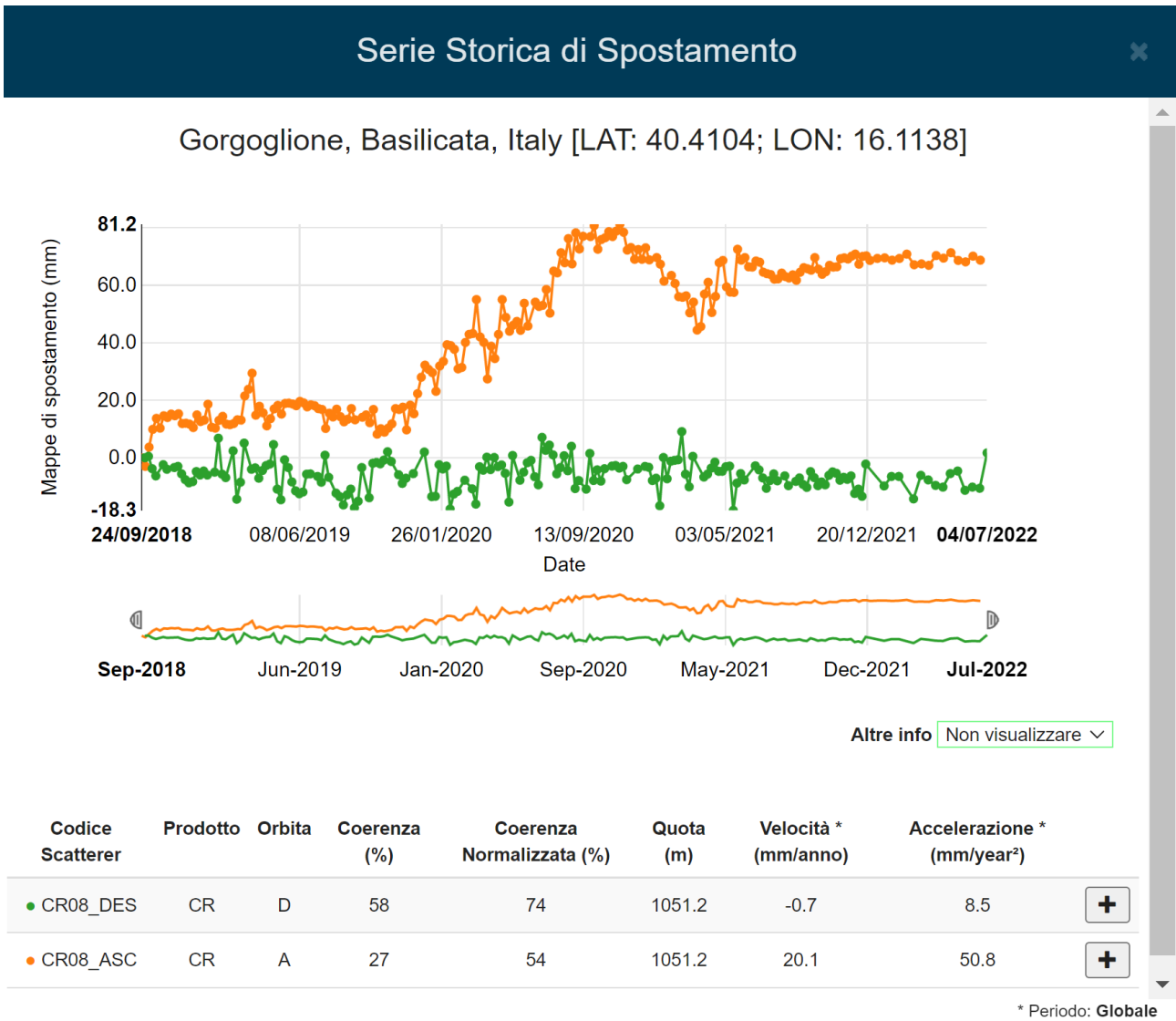
Figura 16: serie temporale di spostamento relativa al periodo settembre 2018 – Giugno 2022 misurata in corrispondenza del Corner Reflector CR08. La serie temporale di spostamento in arancione è relativa all’orbita Ascending mentre quella verde rappresenta la serie temporale relativa all’orbita Descending.
