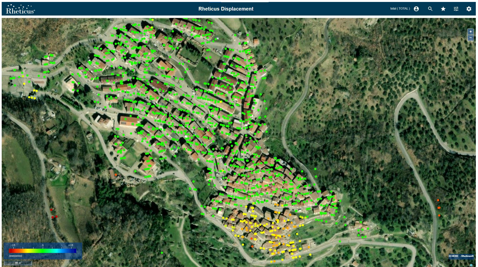
Figura 7: La mappa di velocità media (mm/anno) PS/DS sul centro abitato di Gorgoglione sul periodo esteso a Giugno 2022 non mostra variazioni significative rispetto al precedente rapporto [RD12].
