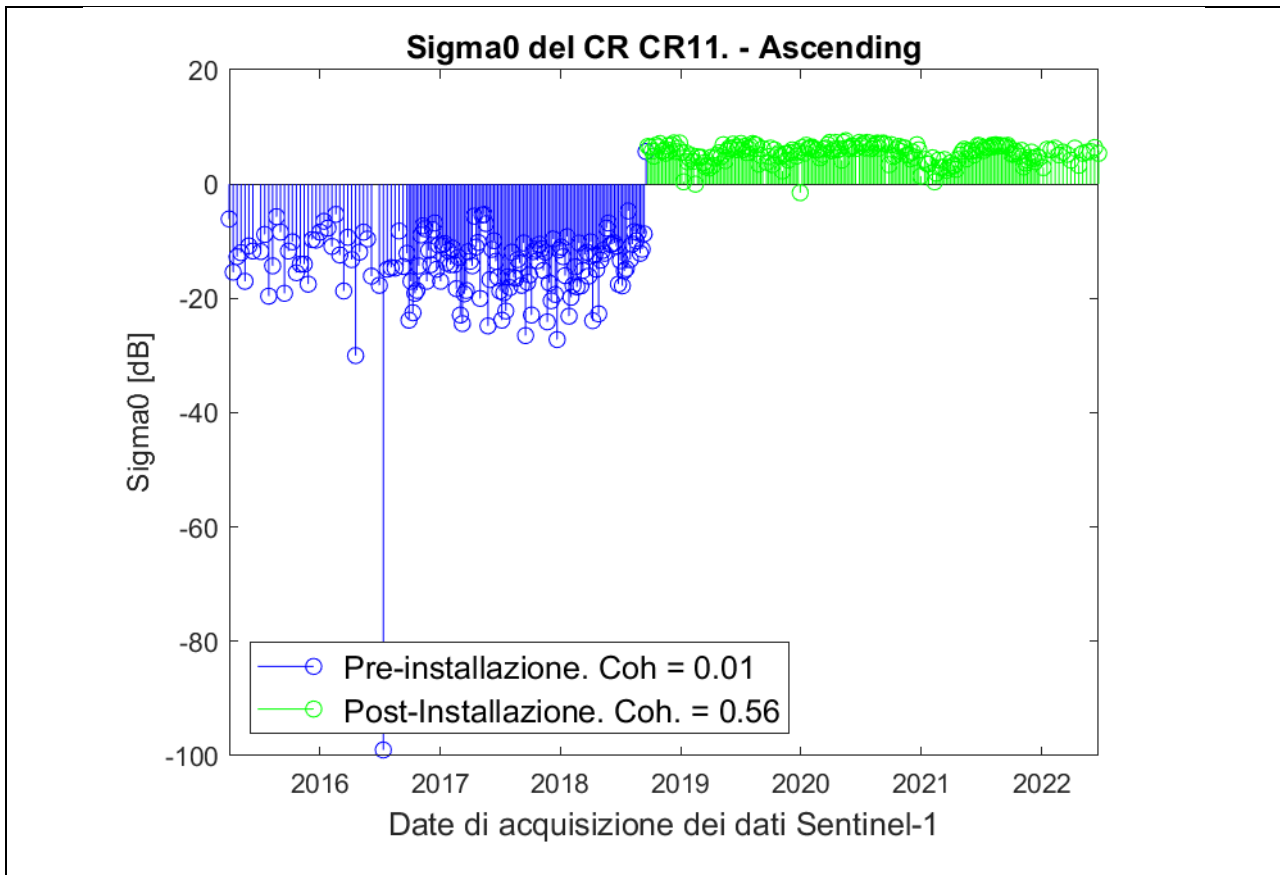
Fig. 0.42: Analisi radiometrica della serie temporale (modalità ascending) in corrispondenza del corner reflector CR11. In blu sono indicate le misure pre-installazione. In verde sono indicate le misure post-installazione.
