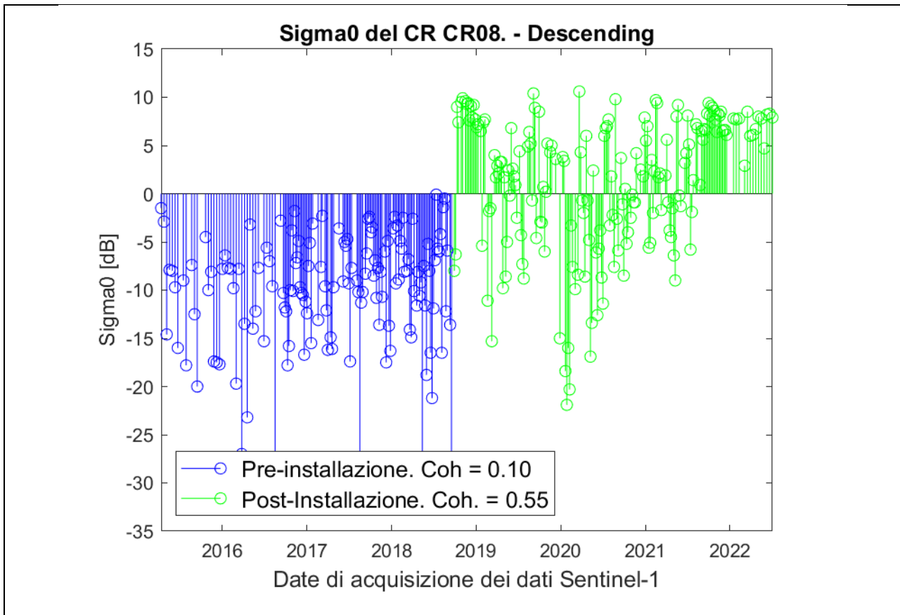
Fig. 0.32: Analisi radiometrica della serie temporale (modalità descending) in corrispondenza del corner reflector CR08. In blu sono indicate le misure pre-installazione. In verde sono indicate le misure post-installazione. Le misure (soprattutto le più recenti) risultano disturbate ed esibiscono valori di sigma0 inferiori ai valori attesi.
