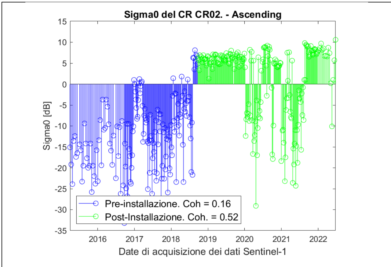
Fig. 0.6: Analisi radiometrica della serie temporale (modalità ascending) in corrispondenza del corner reflector CR02. In blu sono indicate le misure pre-installazione. In verde sono indicate le misure post-installazione.
