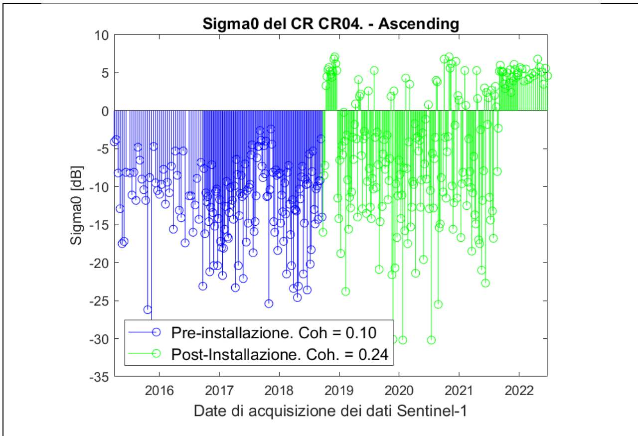
Fig. 0.14: Analisi radiometrica della serie temporale (modalità ascending) in corrispondenza del corner reflector CR04. In blu sono indicate le misure pre-installazione. In verde sono indicate le misure post-installazione. In particolare, la risposta di ampiezza mostra un netto miglioramento dalla risposta del corner a vale delle attività di manutenzione.
