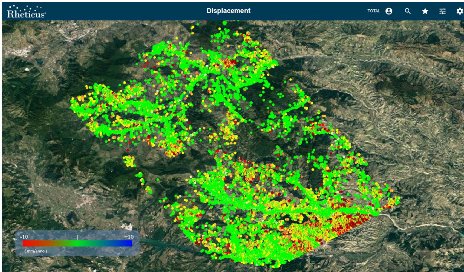
Figura 5: Mappa velocità media annua (mm/anno) lungo la direzione verticale sul periodo esteso a Giugno 2022 ottenuta dalla combinazione delle immagini Ascending e Descending acquisite dal satellite Sentinel-1.
