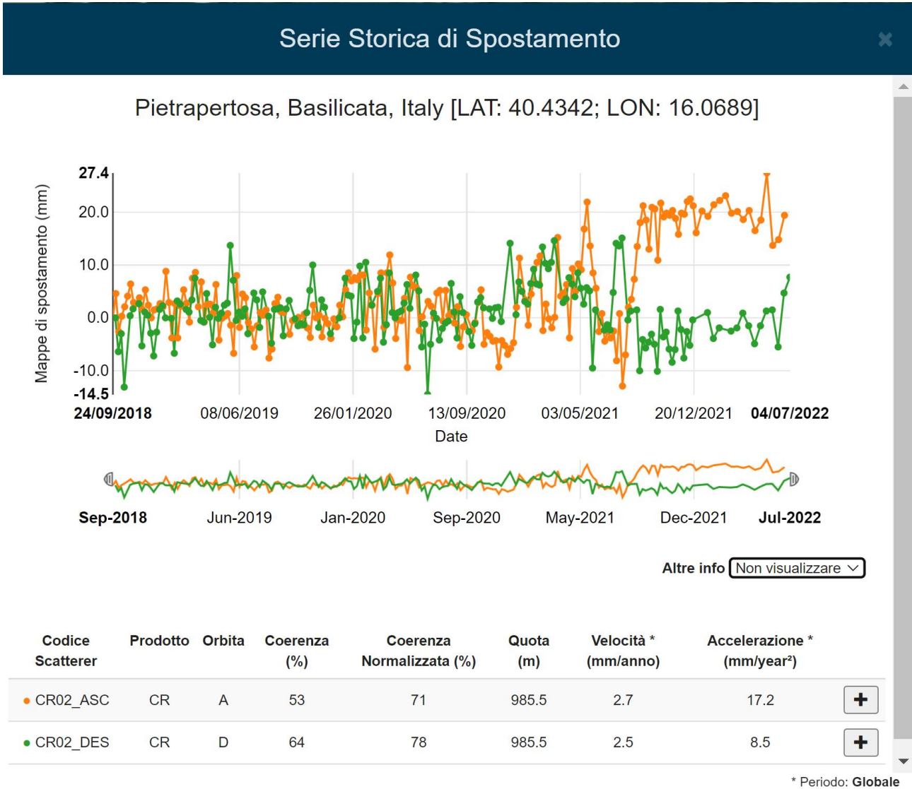
Figura 19: serie temporale di spostamento relativa al periodo settembre 2018 – Giugno 2022 misurata in corrispondenza del Corner Reflector CR02. La serie temporale di spostamento in verde è relativa all'orbita Descending mentre quella arancione rappresenta la serie temporale relativa all'orbita Ascending.
