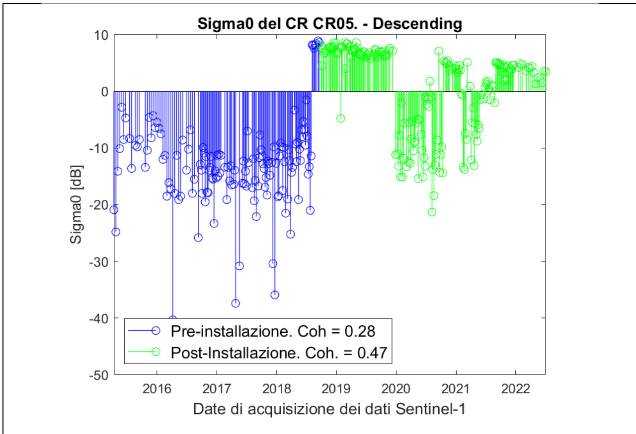
Fig. 0.20: Analisi radiometrica della serie temporale (modalità descending) in corrispondenza del corner reflector CR05. In blu sono indicate le misure pre-installazione. In verde sono indicate le misure post-installazione.
