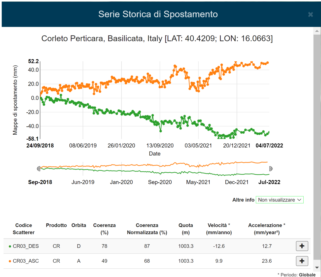
Figura 25: serie temporale di spostamento relativa al periodo settembre 2018 – Giugno 2022 misurata in corrispondenza del Corner Reflector CR03. La serie temporale di spostamento in verde è relativa all'orbita Descending mentre quella arancione rappresenta la serie temporale relativa all'orbita Ascending.
