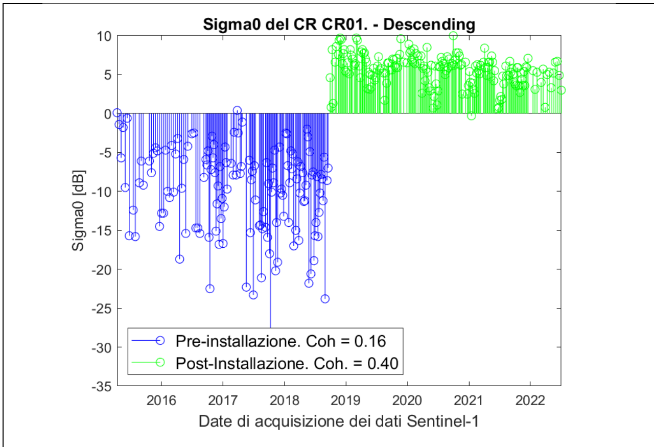
Fig. 0.4: Analisi radiometrica della serie temporale (modalità descending) in corrispondenza del corner reflector CR01. In blu sono indicate le misure pre-installazione. In verde sono indicate le misure post-installazione.
