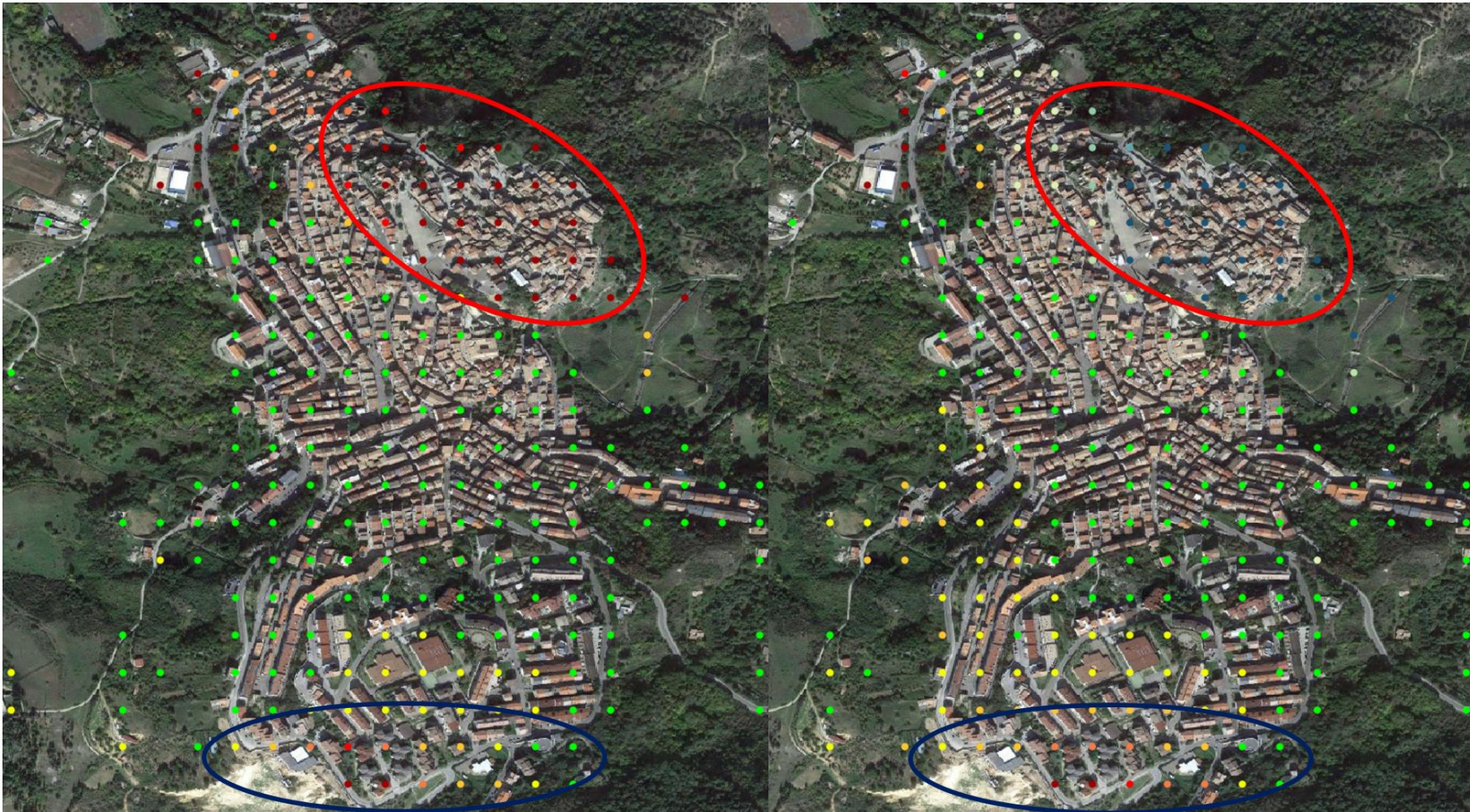
Figura 11: La mappa delle componenti di velocità media Est(+) – Ovest(-) (immagine di sinistra) e Verticale (immagine di destra) sul centro abitato di Stigliano calcolata sul periodo esteso a Giugno 2022 è in linea con quanto misurato nel rapporto precedente [RD12]. Sulla zona nord (evidenziata dal poligono rosso nelle immagini) si evince una velocità media in direzione Est pari a circa 24 mm/anno e una componente di abbassamento verticale medio pari a -15.9 mm/anno mentre la zona sud-ovest (evidenziata dal poligono blu nelle immagini) presenta uno spostamento medio in direzione Ovest pari a -6.6 mm/anno fino ad un massimo di -12.5 mm/anno e una componente di abbassamento verticale media pari a -5.8 mm/anno fino ad un massimo di -11.9 mm/anno.
