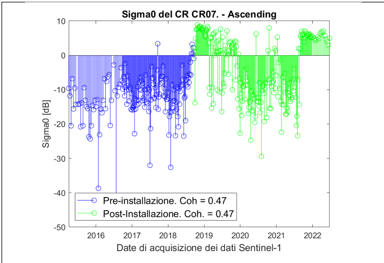
Fig. 0.26: Analisi radiometrica della serie temporale (modalità ascending) in corrispondenza del corner reflector CR07. In blu sono indicate le misure pre-installazione. In verde sono indicate le misure post-installazione. Per alcune date sono evidenti misure rumorose.
