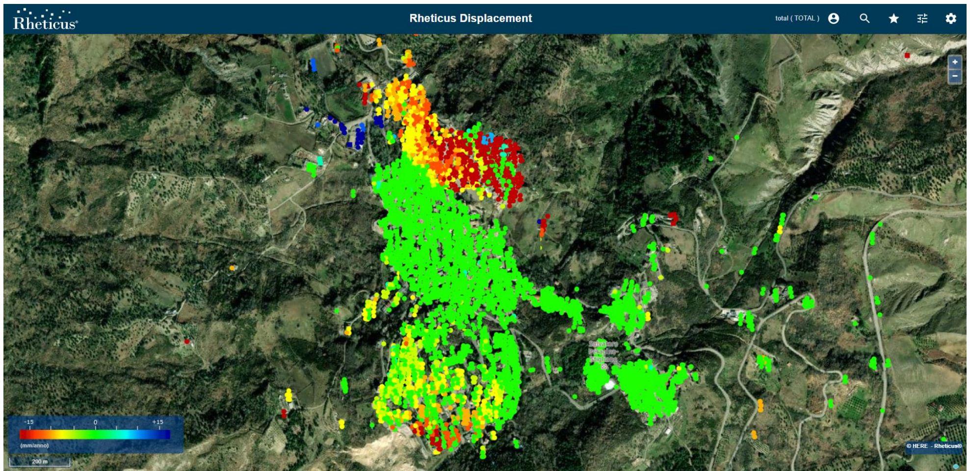
Figura 9: La mappa di velocità media (mm/anno) PS/DS sul centro abitato di Stigliano calcolata sul periodo esteso a Giugno 2022 non mostra variazioni significative rispetto al rapporto precedente [RD12].
