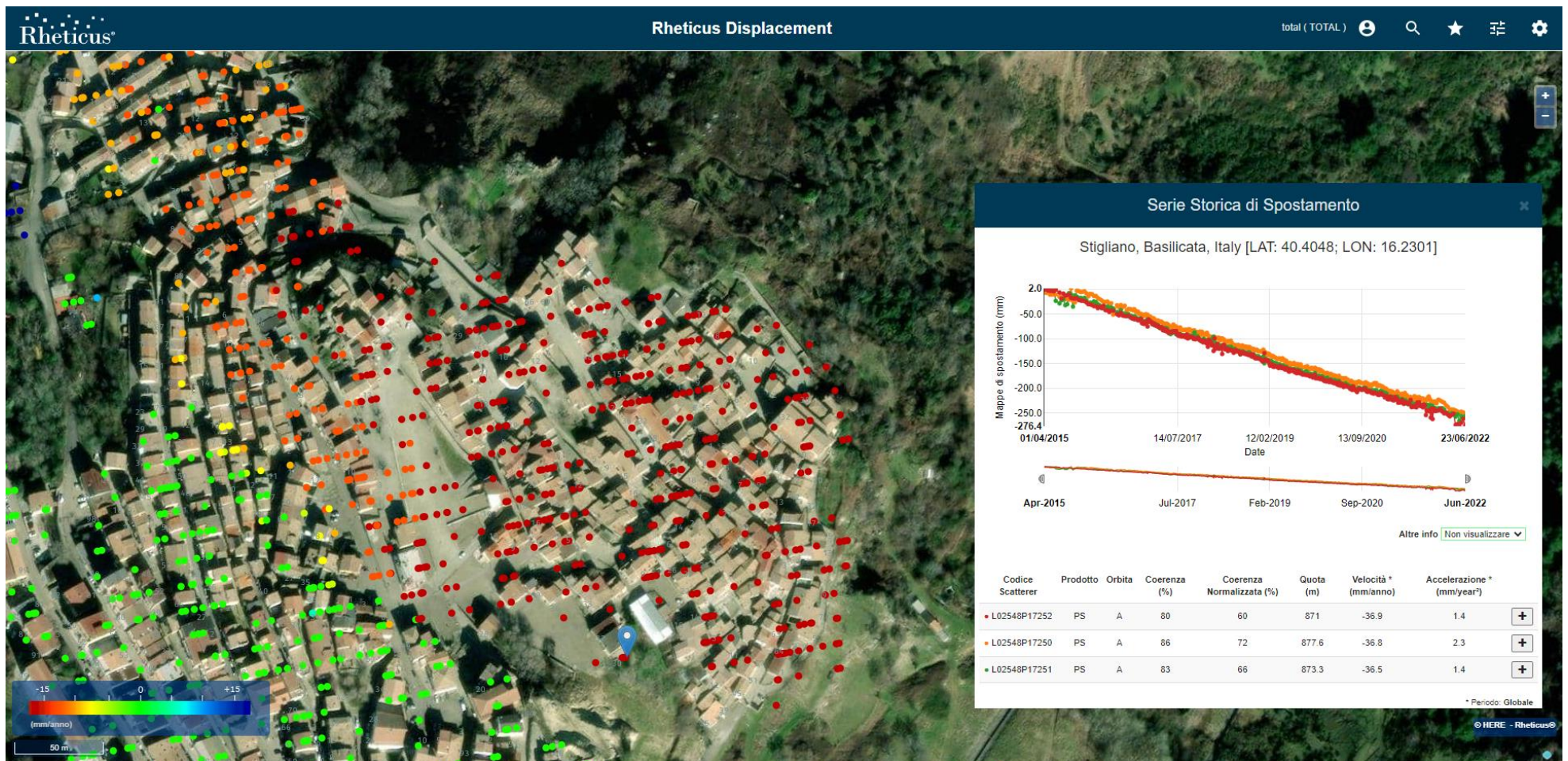
Figura 10: Visualizzazione dei soli PS/DS caratterizzati da una velocità media di abbassamento superiore a -20 mm/anno. Il grafico mostra le serie temporali di 3 PS (evidenziati dal puntatore blu nell'immagine – CODE: L02548P17250, L02548P17251, L02548P17252) a più alta velocità situato nella zona Nord-Est del centro abitato di Stigliano caratterizzato da una velocità media in orbita Ascending pari a circa -37 mm/anno in linea con quanto misurato nel precedente rapporto [RD12].
