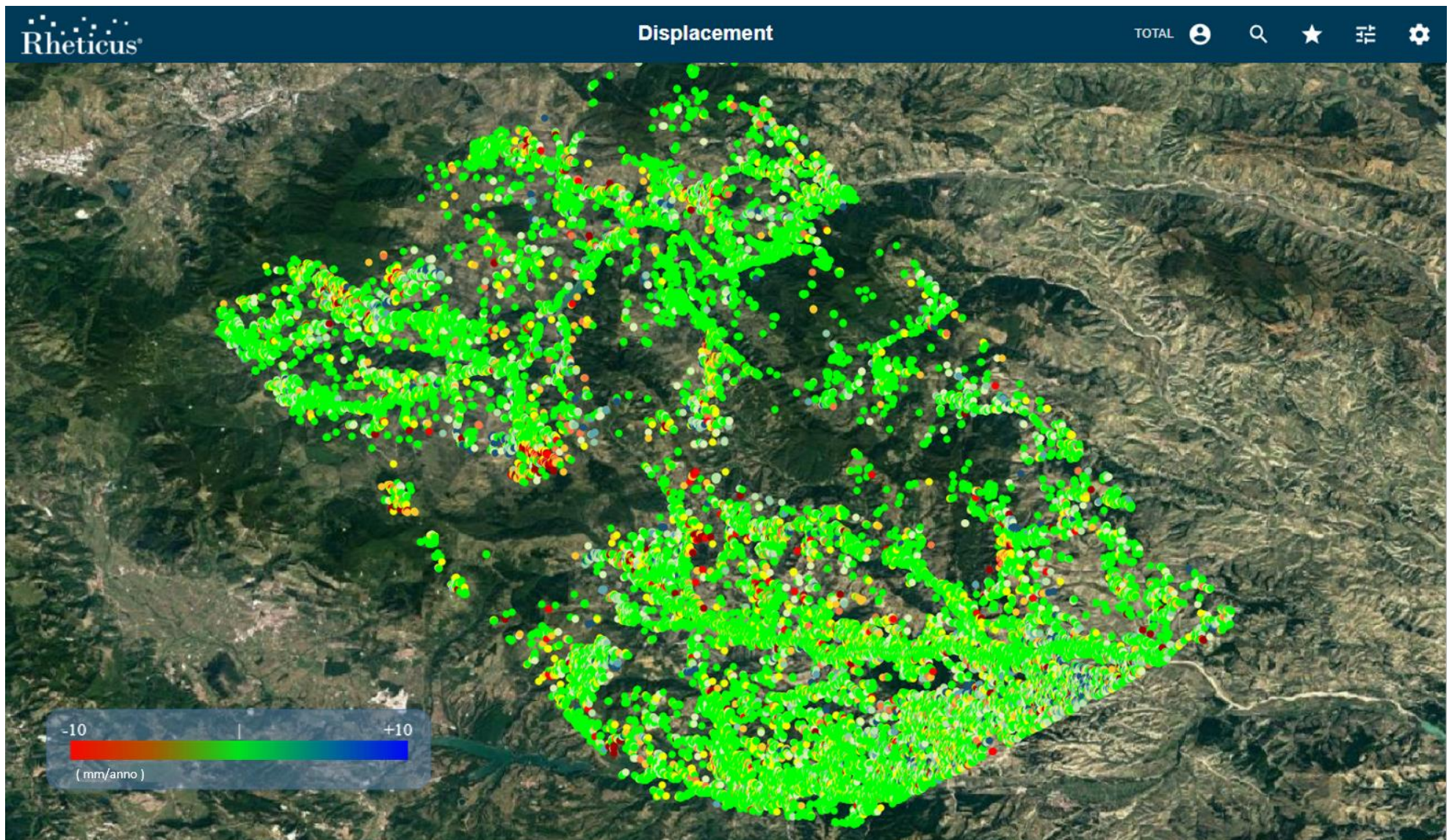
Figura 6: Mappa velocità media annua (mm/anno) in direzione Est(+) - Ovest(-) sul periodo esteso a Giugno 2022 ottenuta dalla combinazione delle immagini Ascending e Descending acquisite dal satellite Sentinel-1.
