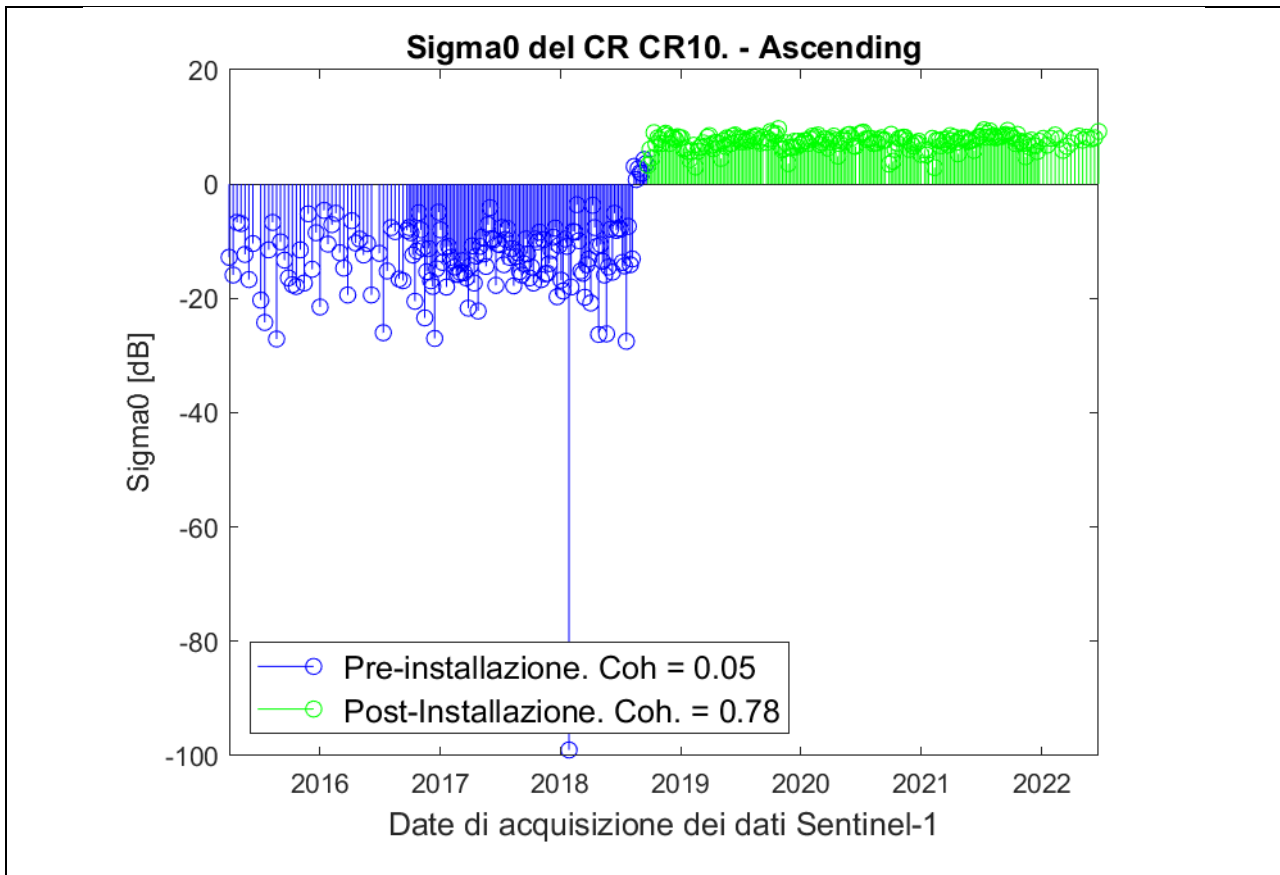
Fig. 0.38: Analisi radiometrica della serie temporale (modalità ascending) in corrispondenza del corner reflector CR10. In blu sono indicate le misure pre-installazione. In verde sono indicate le misure post-installazione.
