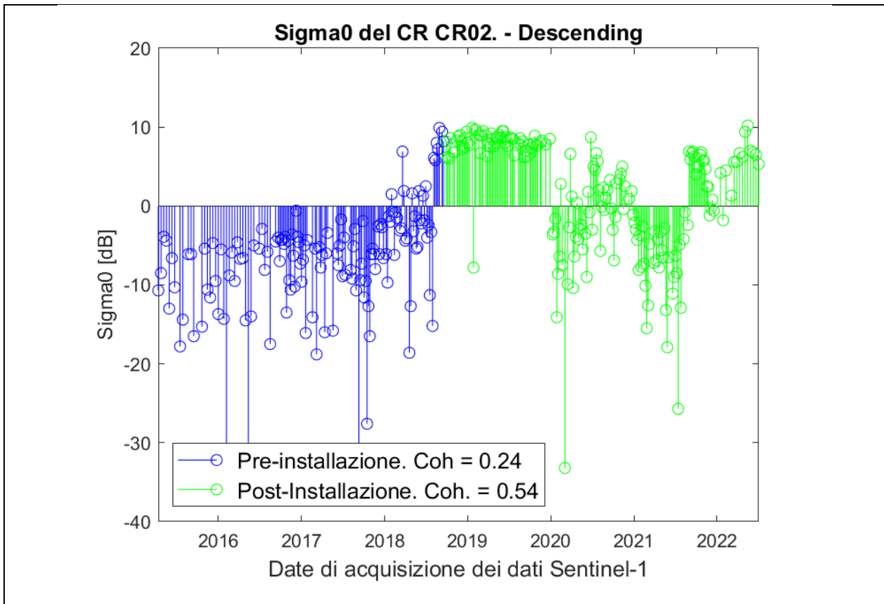
Fig. 0.8: Analisi radiometrica della serie temporale (modalità descending) in corrispondenza del corner reflector CR02. In blu sono indicate le misure pre-installazione. In verde sono indicate le misure post-installazione.
