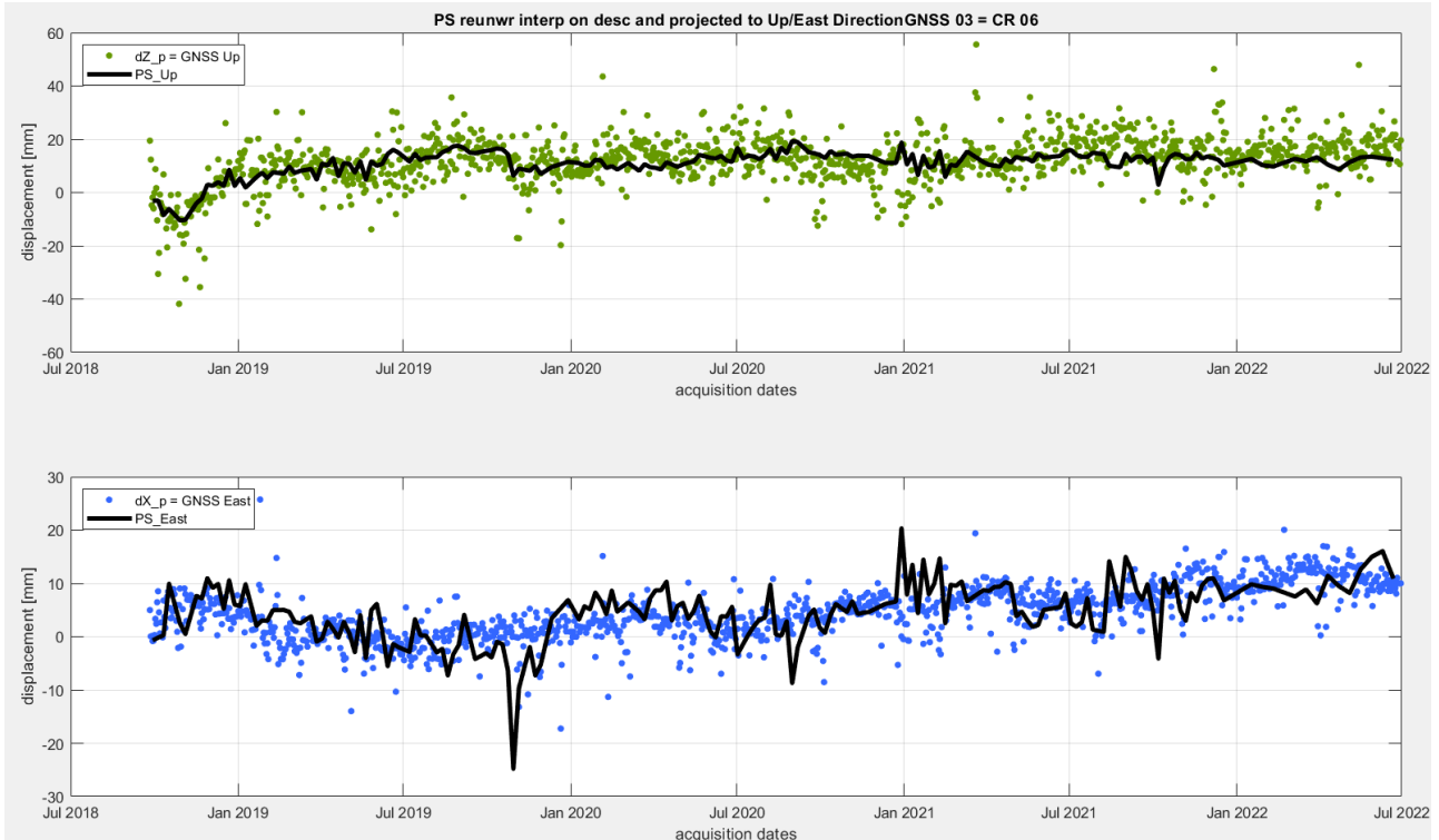
Figura 44: la figura in alto riporta la proiezione delle misure SAR in corrispondenza del Corner Reflector CR06 in direzione verticale (linea nera) unitamente alle misure di spostamento verticale GNSS (punti verdi) mentre la figura in basso riporta la proiezione delle misure SAR in direzione est (linea nera) unitamente alle misure GNSS nella stessa direzione (punti blu). Si nota un ottimo accordo a livello qualitativo.
