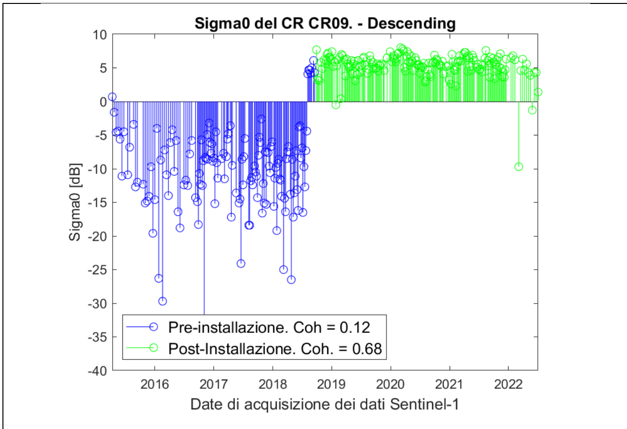
Fig. 0.36: Analisi radometrica della serie temporale (modalità descending) in corrispondenza del corner reflector CR09. In blu sono indicate le misure pre-installazione. In verde sono indicate le misure post-installazione.
