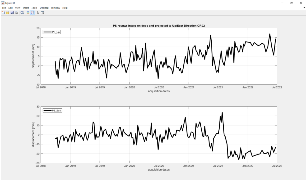
Figura 20: il grafico in alto rappresenta la serie temporale di spostamento in direzione Verticale (PS_Up) mentre il grafico in basso rappresenta la serie temporale di spostamento in direzione est (PS_Est).
