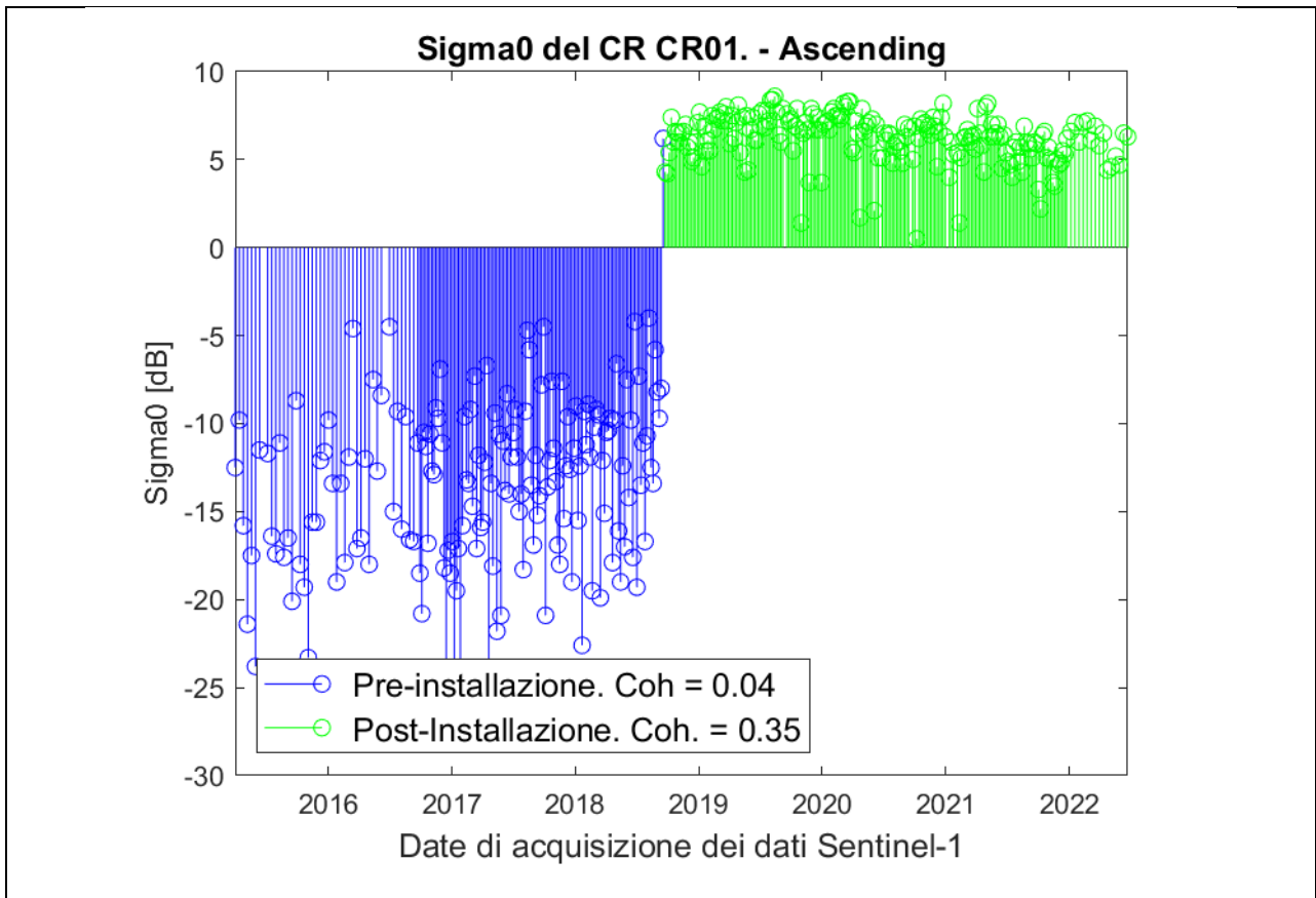
Fig. 0.2: Analisi radiometrica della serie temporale (modalità ascending) in corrispondenza del corner reflector CR01. In blu sono indicate le misure pre-installazione. In verde sono indicate le misure post-installazione.
