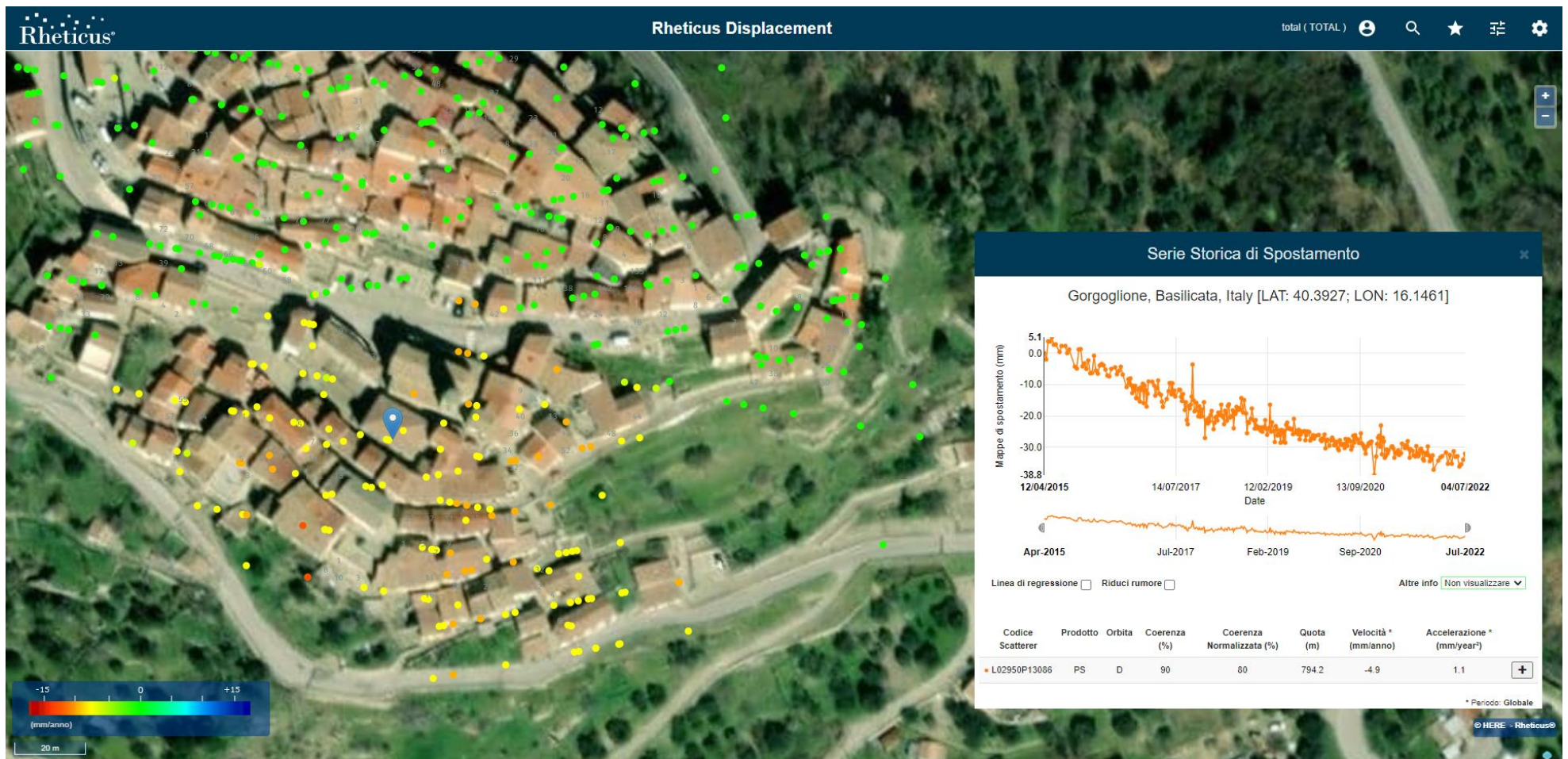
Figura 8: Serie temporale del PS (evidenziato dal puntatore blu nell'immagine) ad alta coerenza (0.90) situato al centro dell'area in movimento del centro abitato di Gorgoglione . La velocità media del PS sul periodo esteso a Giugno 2022 è pari a -4.9 mm/anno in linea con quanto misurato nel precedente rapporto [RD12].
