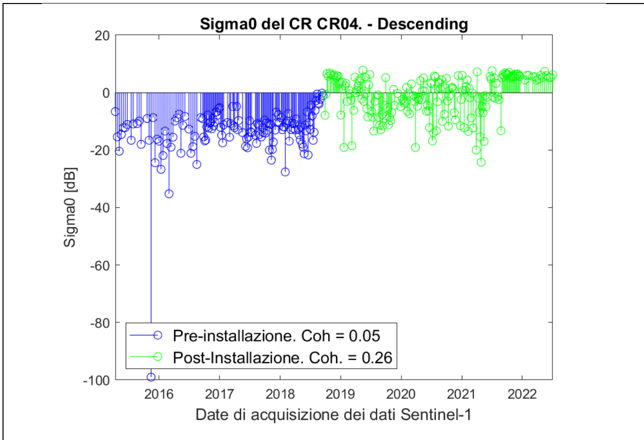
Fig. 0.16: Analisi radiometrica della serie temporale (modalità descending) in corrispondenza del corner reflector CR04. In blu sono indicate le misure pre-installazione. In verde sono indicate le misure post-installazione. Una corretta installazione del corner dovrebbe fare apprezzare nella fase di post-installazione un segnale con maggiore intensità. In questo caso la risposta di ampiezza esibisce una notevole variabilità.
