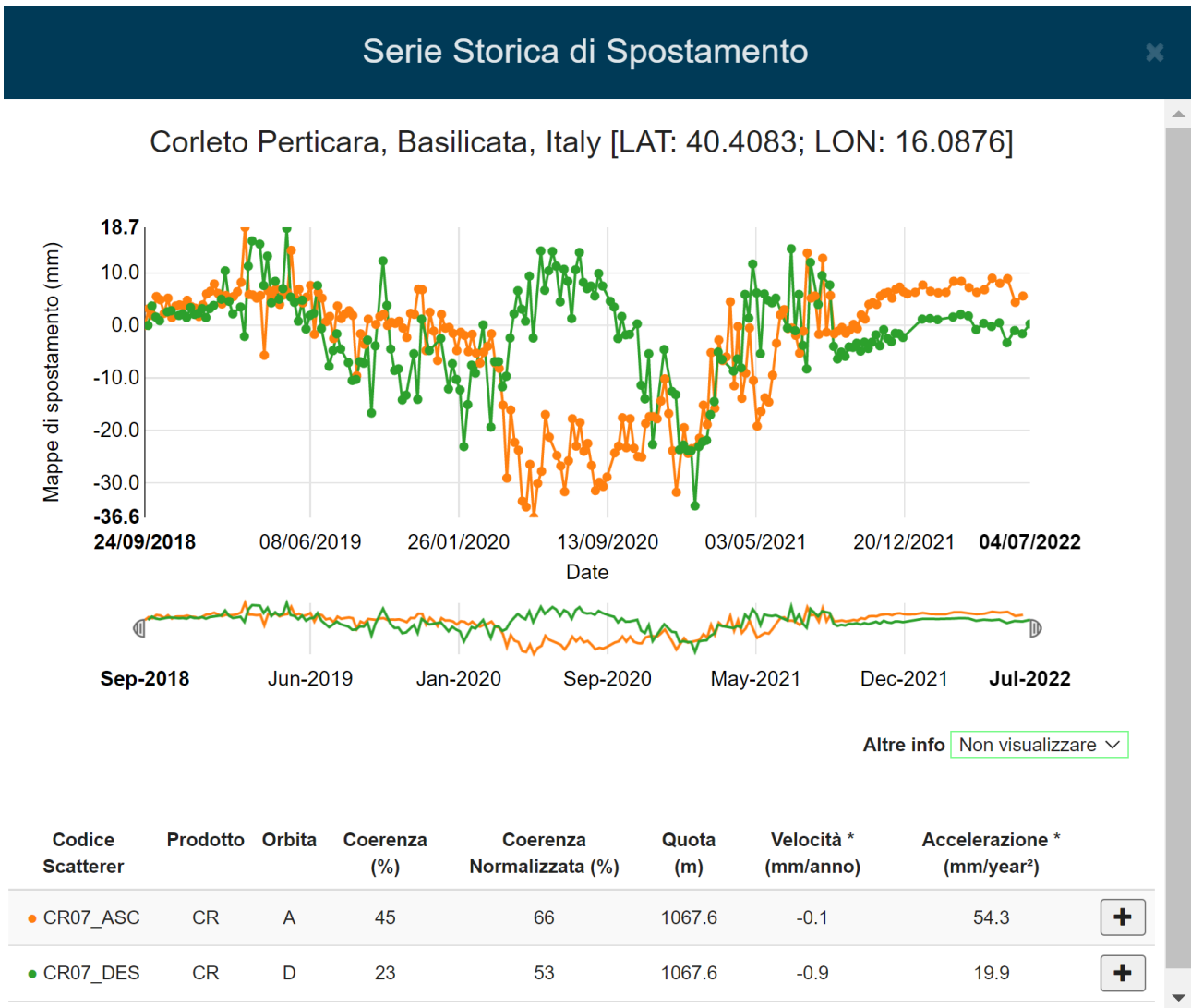
Figura 34: serie temporale di spostamento relativa al periodo settembre 2018 – Giugno 2022 misurata in corrispondenza del Corner Reflector CR07. La serie temporale di spostamento in verde è relativa all'orbita Descending mentre quella arancione rappresenta la serie temporale relativa all'orbita Ascending.
