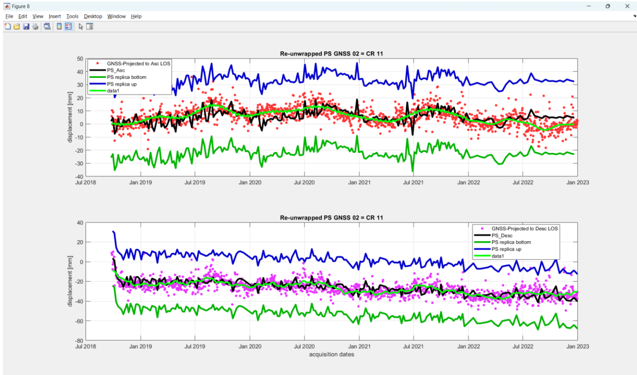
Figura 40: la figura in alto riporta la proiezione delle misure GNSS in corrispondenza del Corner Reflector CR11 (punti rossi) sulla viste SAR ascending mentre la figura in basso riporta la proiezione delle misure GNSS sulla vista SAR descending (punti viola) e raffronto con le misure SAR rappresentate dalla linea nera (le linee blu e verdi rappresentano le due repliche delle misure SAR di una quantità pari a \pm \lambda/2 ). Si nota un ottimo accordo a livello qualitativo.
