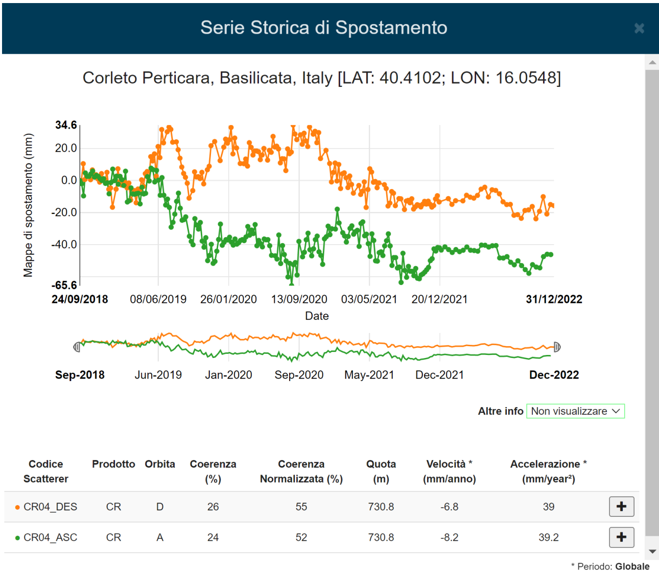
Figura 22: serie temporale di spostamento relativa al periodo settembre 2018 – Dicembre 2022 misurata in corrispondenza del Corner Reflector CR04. La serie temporale di spostamento in verde è relativa all’orbita Ascending mentre quella arancione rappresenta la serie temporale relativa all’orbita Descending.
