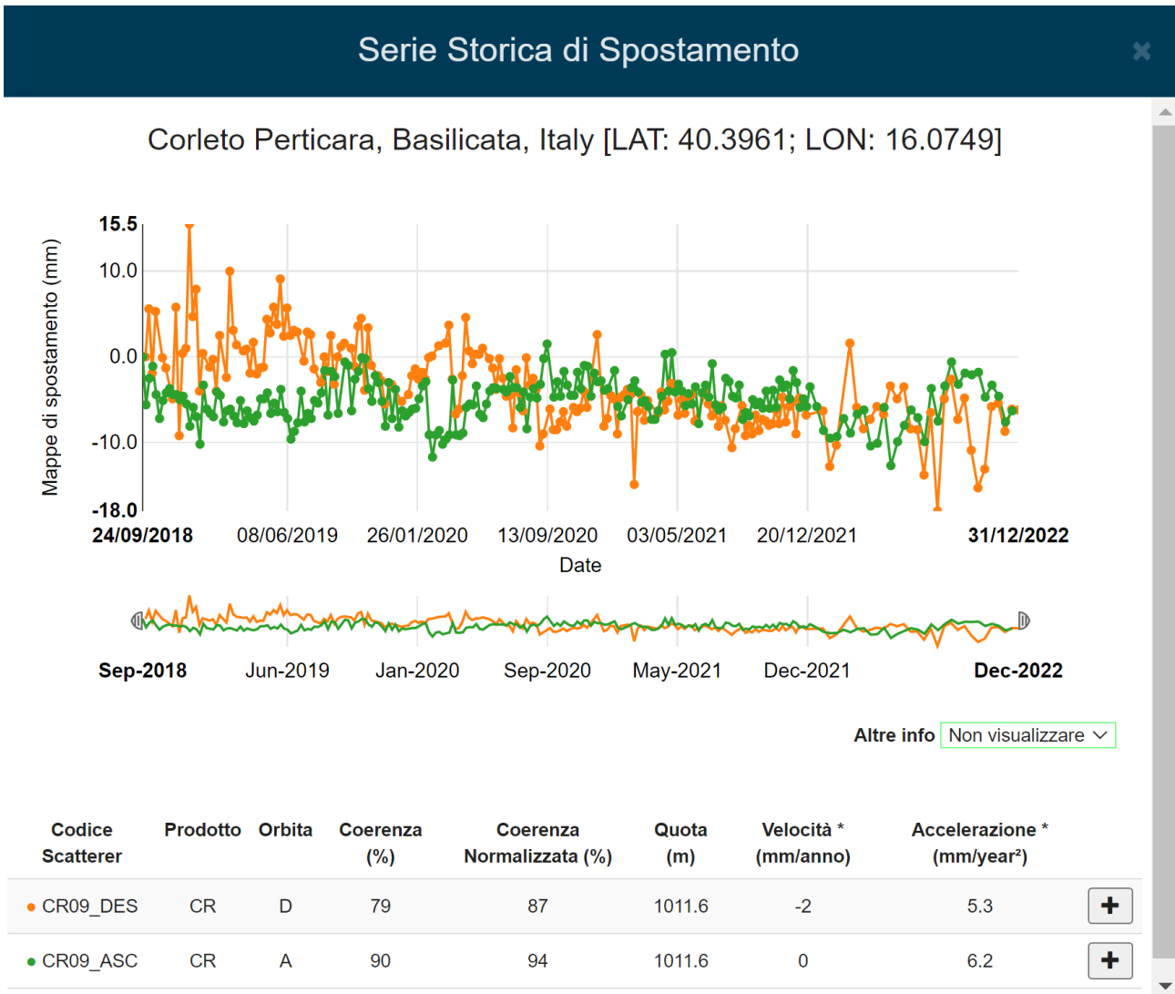
Figura 28: serie temporale di spostamento relativa al periodo settembre 2018 – Dicembre 2022 misurata in corrispondenza del Corner Reflector CR09. La serie temporale di spostamento in verde è relativa all’orbita Ascending mentre quella arancione rappresenta la serie temporale relativa all’orbita Descending.
