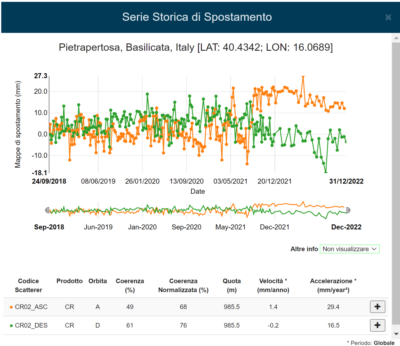
Figura 19: serie temporale di spostamento relativa al periodo settembre 2018 – Dicembre 2022 misurata in corrispondenza del Corner Reflector CR02. La serie temporale di spostamento in verde è relativa all'orbita Descending mentre quella arancione rappresenta la serie temporale relativa all'orbita Ascending.
