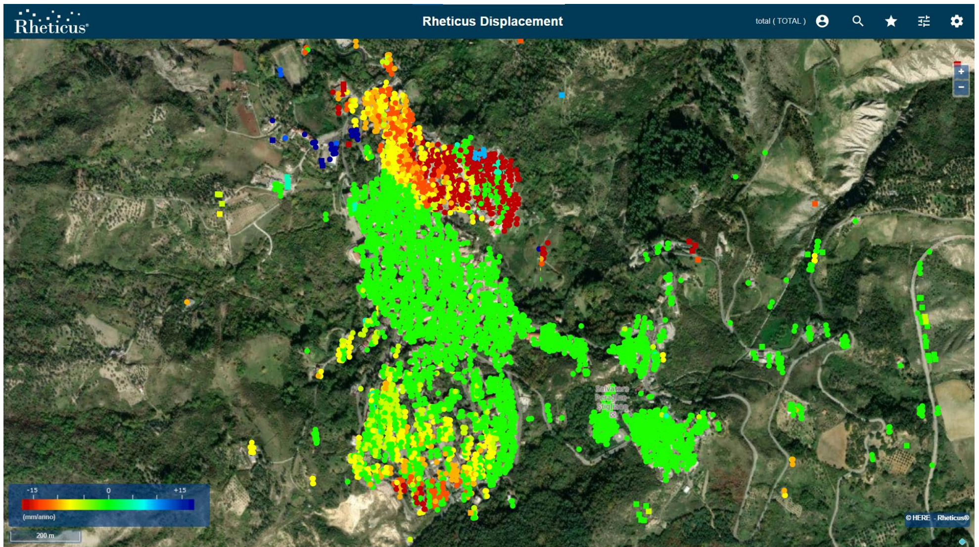
Figura 9: La mappa di velocità media (mm/anno) PS/DS sul centro abitato di Stigliano calcolata sul periodo esteso a Dicembre 2022 non mostra variazioni significative rispetto al rapporto precedente [RD13].
