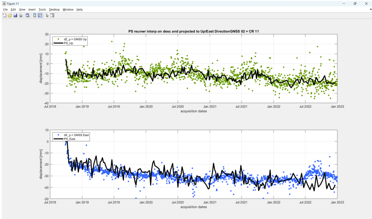
Figura 43: la figura in alto riporta la proiezione delle misure SAR in corrispondenza del Corner Reflector CR11 in direzione verticale (linea nera) unitamente alle misure di spostamento verticale GNSS (punti verdi) mentre la figura in basso riporta la proiezione delle misure SAR in direzione est (linea nera) unitamente alle misure GNSS nella stessa direzione (punti blu). Si nota un ottimo accordo a livello qualitativo.
