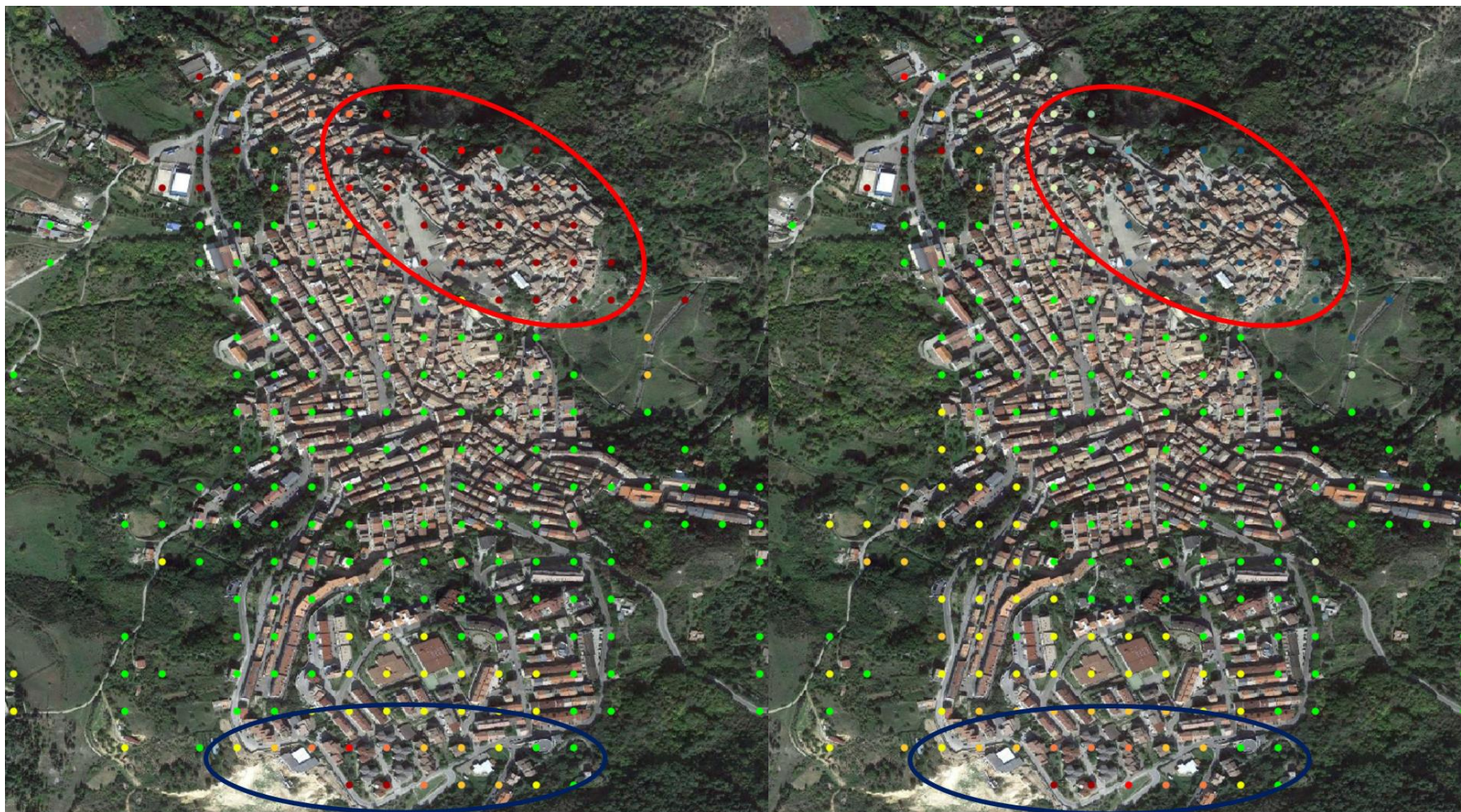
Figura 11: La mappa delle componenti di velocità media Est(+) – Ovest(-) (immagine di sinistra) e Verticale (immagine di destra) sul centro abitato di Stigliano calcolata sul periodo esteso a Dicembre 2022 è in linea con quanto misurato nel rapporto precedente [RD13]. Sulla zona nord (evidenziata dal poligono rosso nelle immagini) si evince una velocità media in direzione Est pari a circa 24 mm/anno e una componente di abbassamento verticale medio pari a -15.3 mm/anno mentre la zona sud-ovest (evidenziata dal poligono blu nelle immagini) presenta uno spostamento medio in direzione Ovest pari a -6.7 mm/anno fino ad un massimo di -14.5 mm/anno e una componente di abbassamento verticale media pari a -5.2 mm/anno fino ad un massimo di -14.0 mm/anno.
