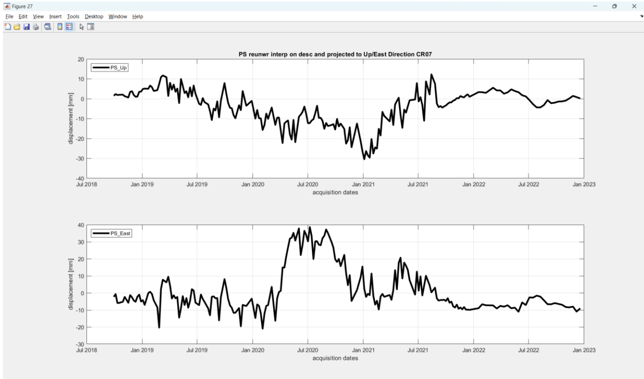
Figura 35: il grafico in alto rappresenta la serie temporale di spostamento in direzione Verticale (PS_Up) mentre il grafico in basso rappresenta la serie temporale di spostamento in direzione est (PS_Est).
