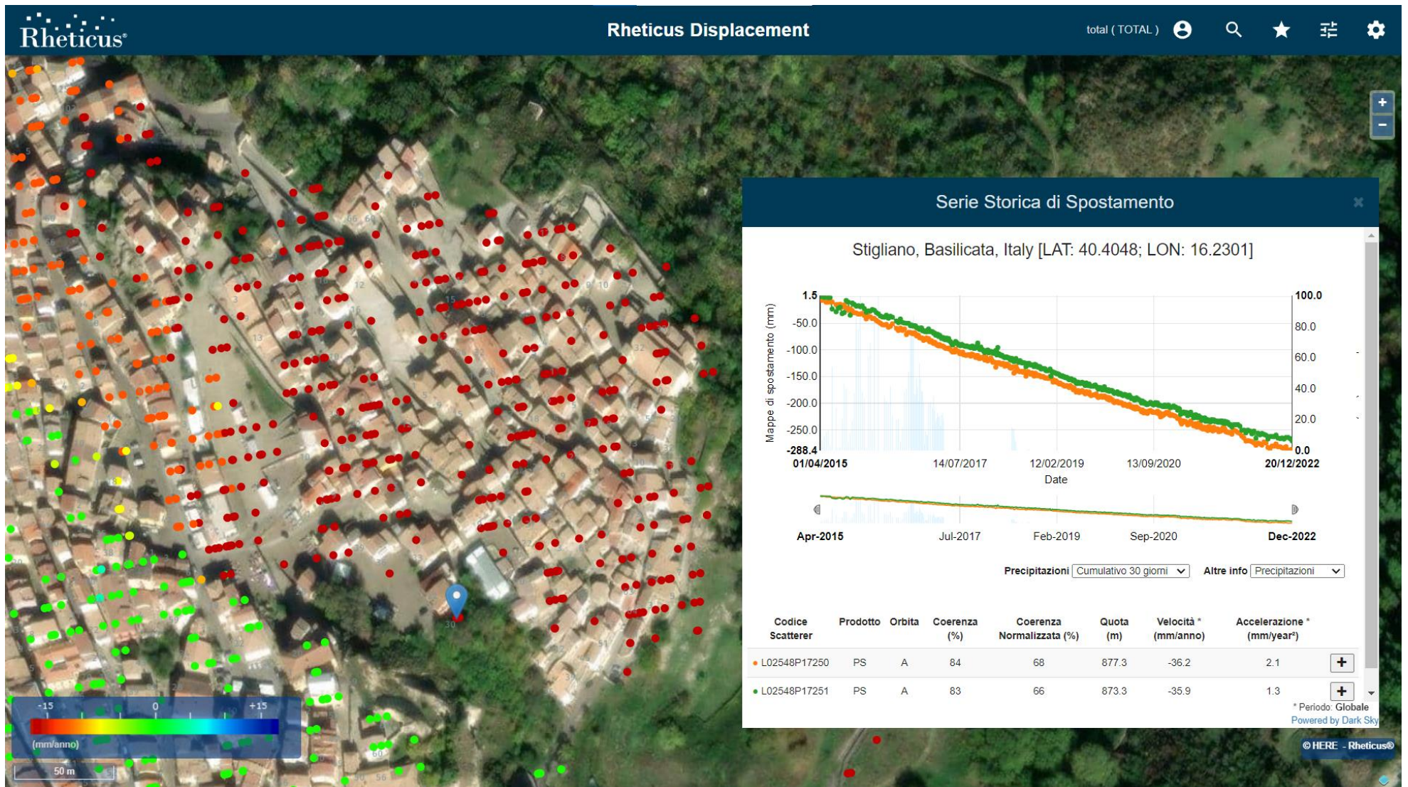
Figura 10: Visualizzazione dei soli PS/DS caratterizzati da una velocità media di abbassamento superiore a -20 mm/anno. Il grafico mostra le serie temporali di 3 PS (evidenziati dal puntatore blu nell'immagine – CODE: L02548P17250, L02548P17251) a più alta velocità situato nella zona Nord-Est del centro abitato di Stigliano caratterizzato da una velocità media in orbita Ascending pari a circa -36 mm/anno in linea con quanto misurato nel precedente rapporto [RD13].
