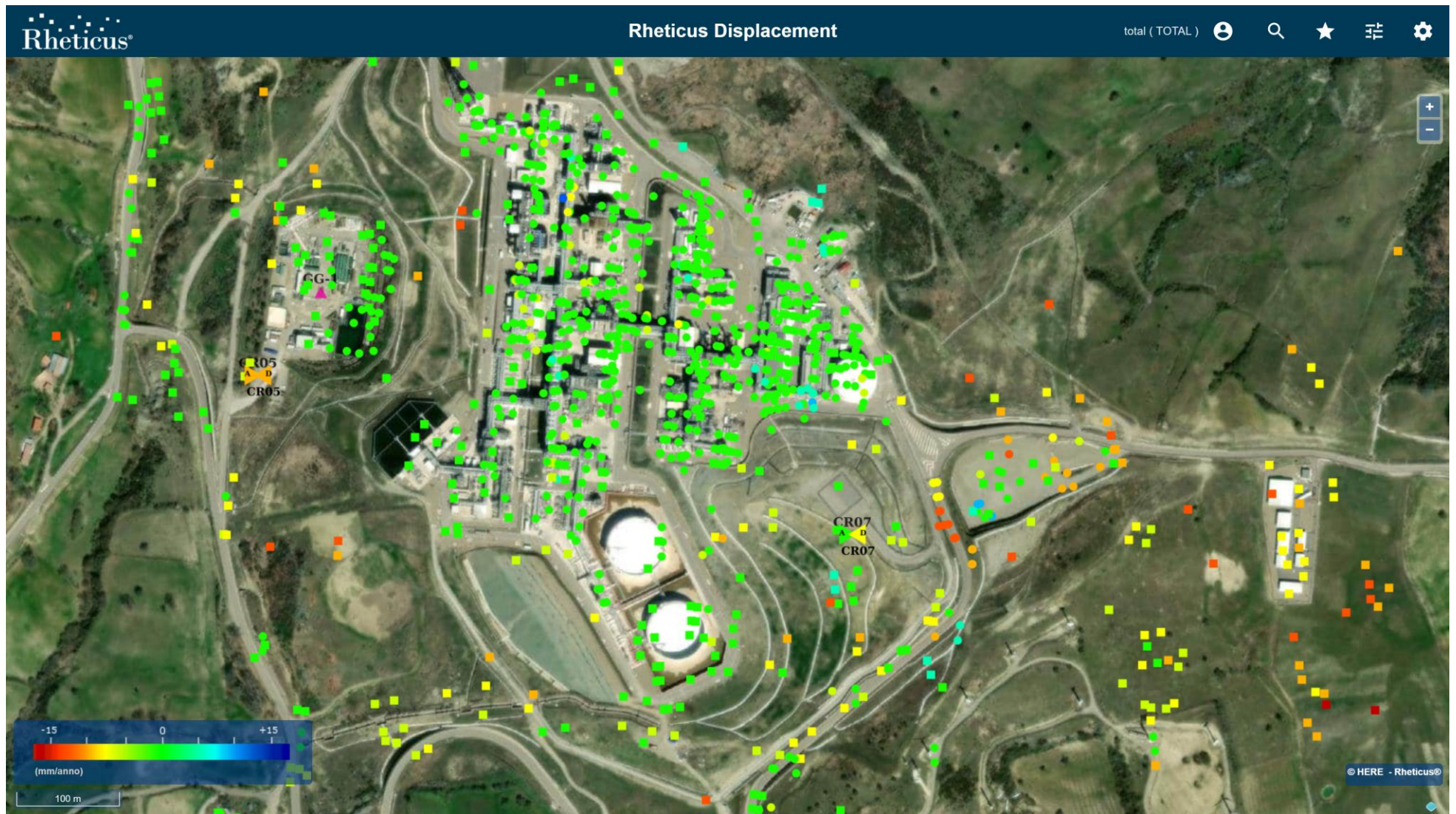
Figura 33: Oil Center caratterizzato da una buona copertura di PS e dai quali nel periodo esteso a Dicembre 2022, non si evincono variazioni significative di velocità media rispetto al precedente rapporto [RD13].
