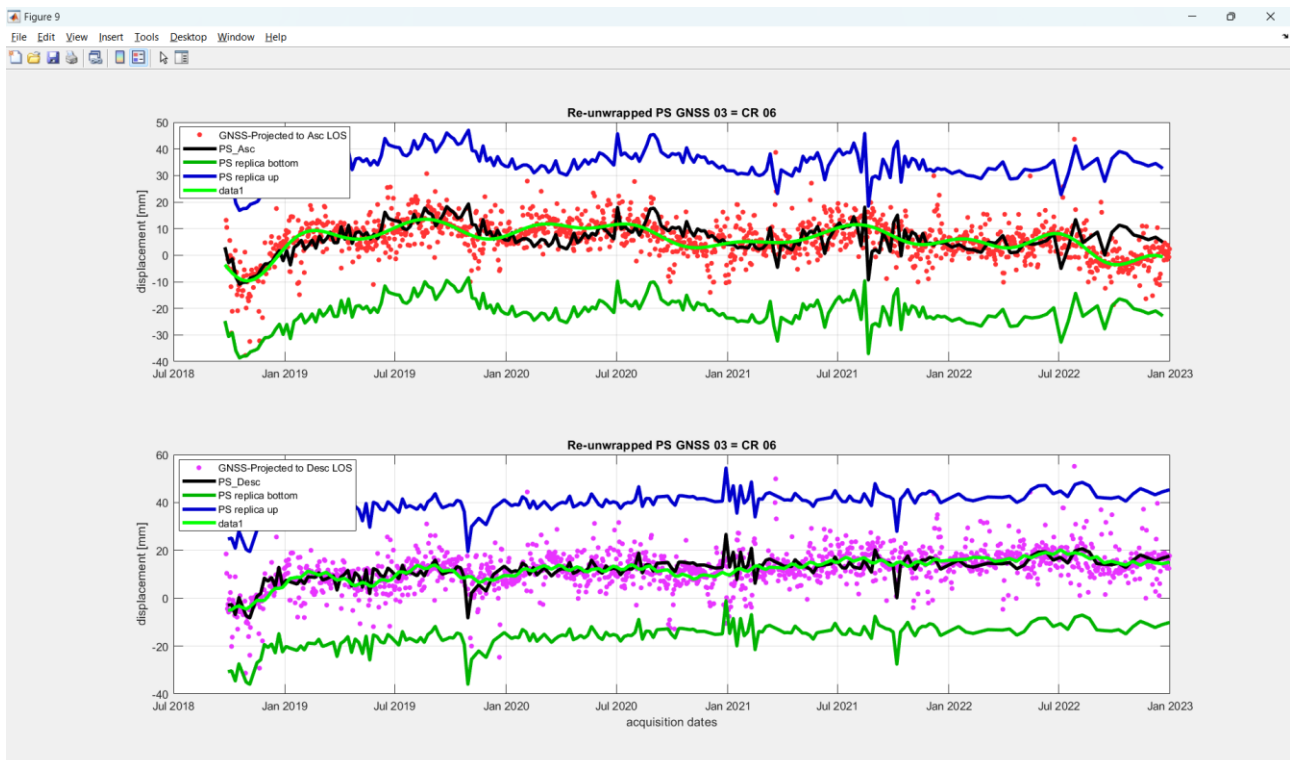
Figura 41: la figura in alto riporta la proiezione delle misure GNSS in corrispondenza del Corner Reflector CR06 (punti rossi) sulla viste SAR ascending mentre la figura in basso riporta la proiezione delle misure GNSS sulla vista SAR descending (punti viola) e raffronto con le misure SAR rappresentate dalla linea nera (le linee blu e verdi rappresentano le due repliche delle misure SAR di una quantità pari a \pm \lambda/2 ). Si nota un ottimo accordo a livello qualitativo.
