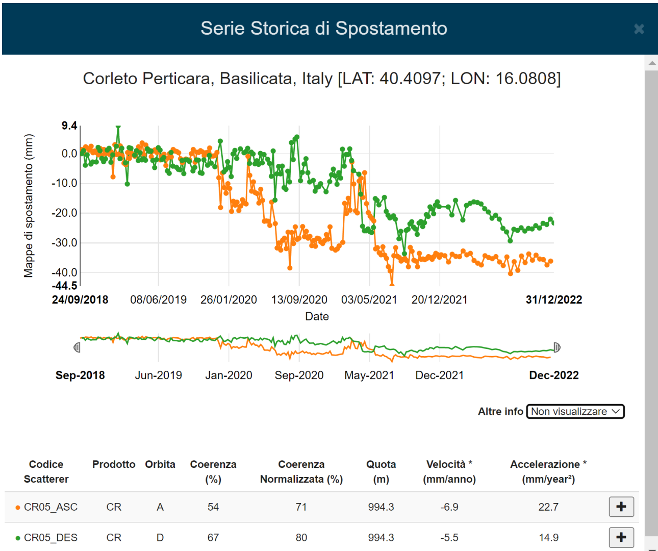
Figura 13: serie temporale di spostamento relativa al periodo settembre 2018 – dicembre 2022 misurata in corrispondenza del Corner Reflector CR05. La serie temporale di spostamento in arancione è relativa all'orbita Ascending mentre quella verde rappresenta la serie temporale relativa all'orbita Descending.
