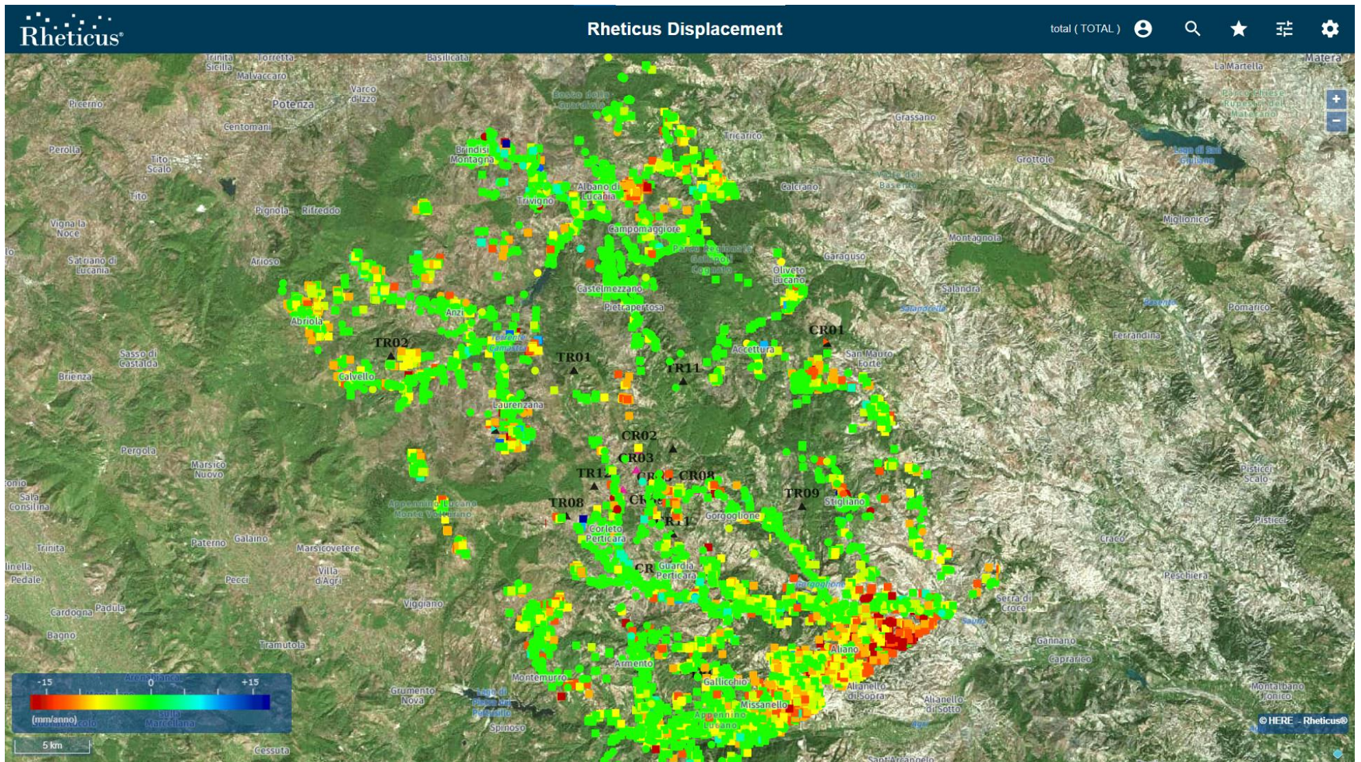
Figura 3: Mappa velocità media annua (mm/anno) lungo la LOS sul periodo esteso a Dicembre 2022 ottenuta dal processamento del dataset Sentinel-1 in orbita ascending.
