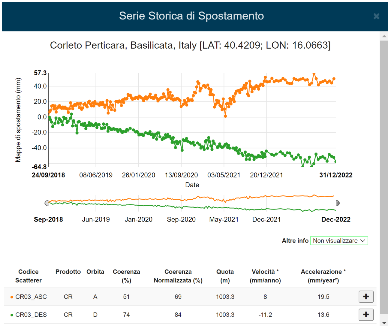
Figura 25: serie temporale di spostamento relativa al periodo settembre 2018 – Dicembre 2022 misurata in corrispondenza del Corner Reflector CR03. La serie temporale di spostamento in verde è relativa all'orbita Descending mentre quella arancione rappresenta la serie temporale relativa all'orbita Ascending.
