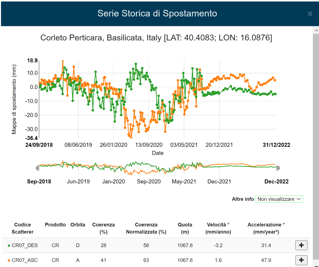
Figura 34: serie temporale di spostamento relativa al periodo settembre 2018 – Dicembre 2022 misurata in corrispondenza del Corner Reflector CR07. La serie temporale di spostamento in verde è relativa all'orbita Descending mentre quella arancione rappresenta la serie temporale relativa all'orbita Ascending.
