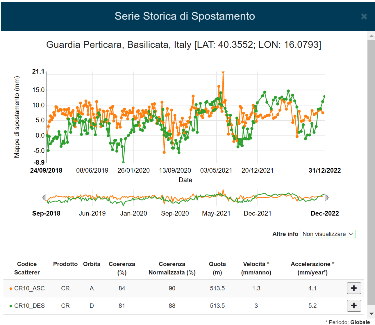
Figura 31: serie temporale di spostamento relativa al periodo settembre 2018 – Dicembre 2022 misurata in corrispondenza del Corner Reflector CR10. La serie temporale di spostamento in verde è relativa all'orbita Descending mentre quella arancione rappresenta la serie temporale relativa all'orbita Ascending.
