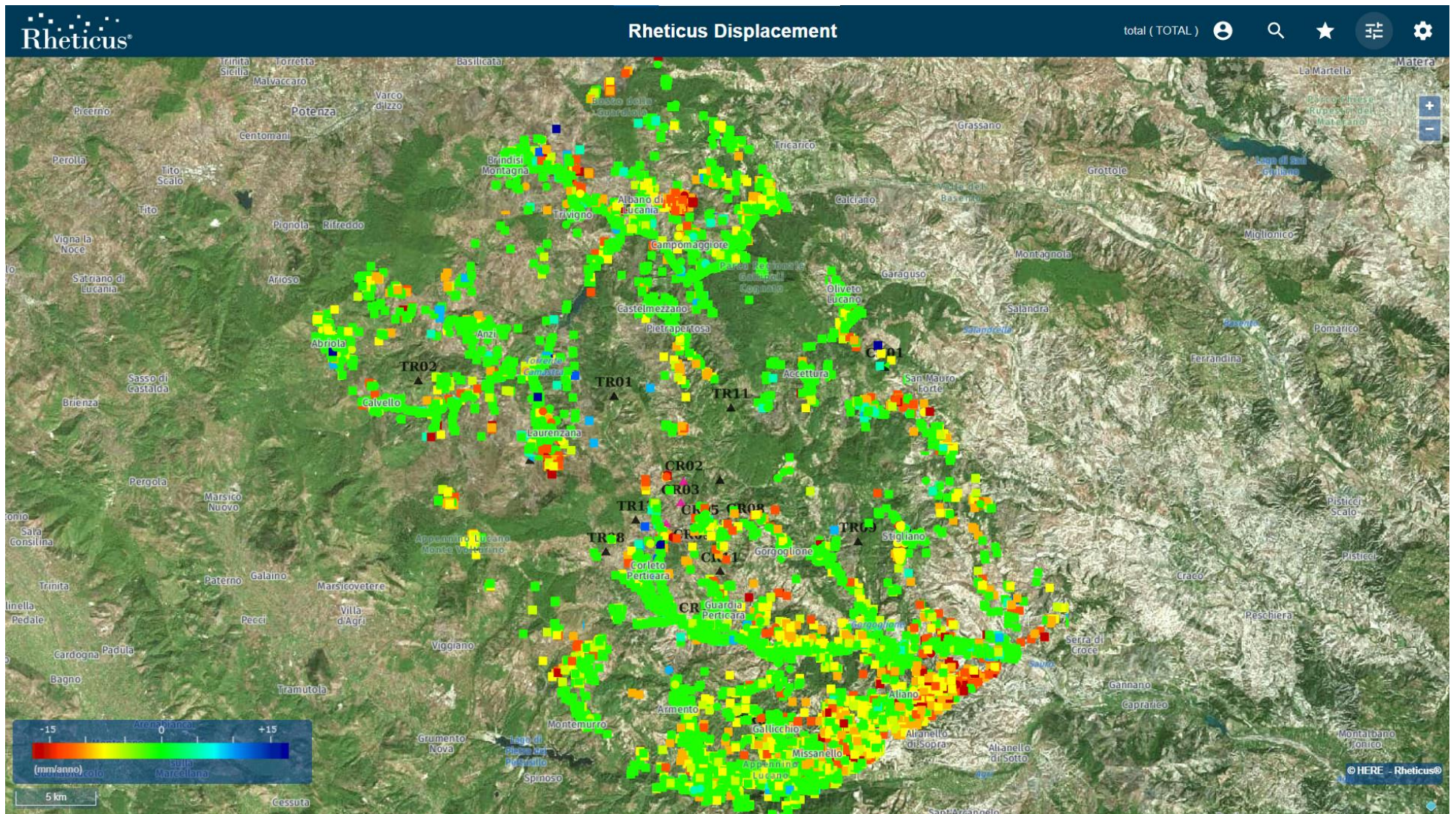
Figura 4: Mappa velocità media annua (mm/anno) lungo la LOS sul periodo esteso a Dicembre 2022 ottenuta dal processamento del dataset Sentinel-1 in orbita descending.
