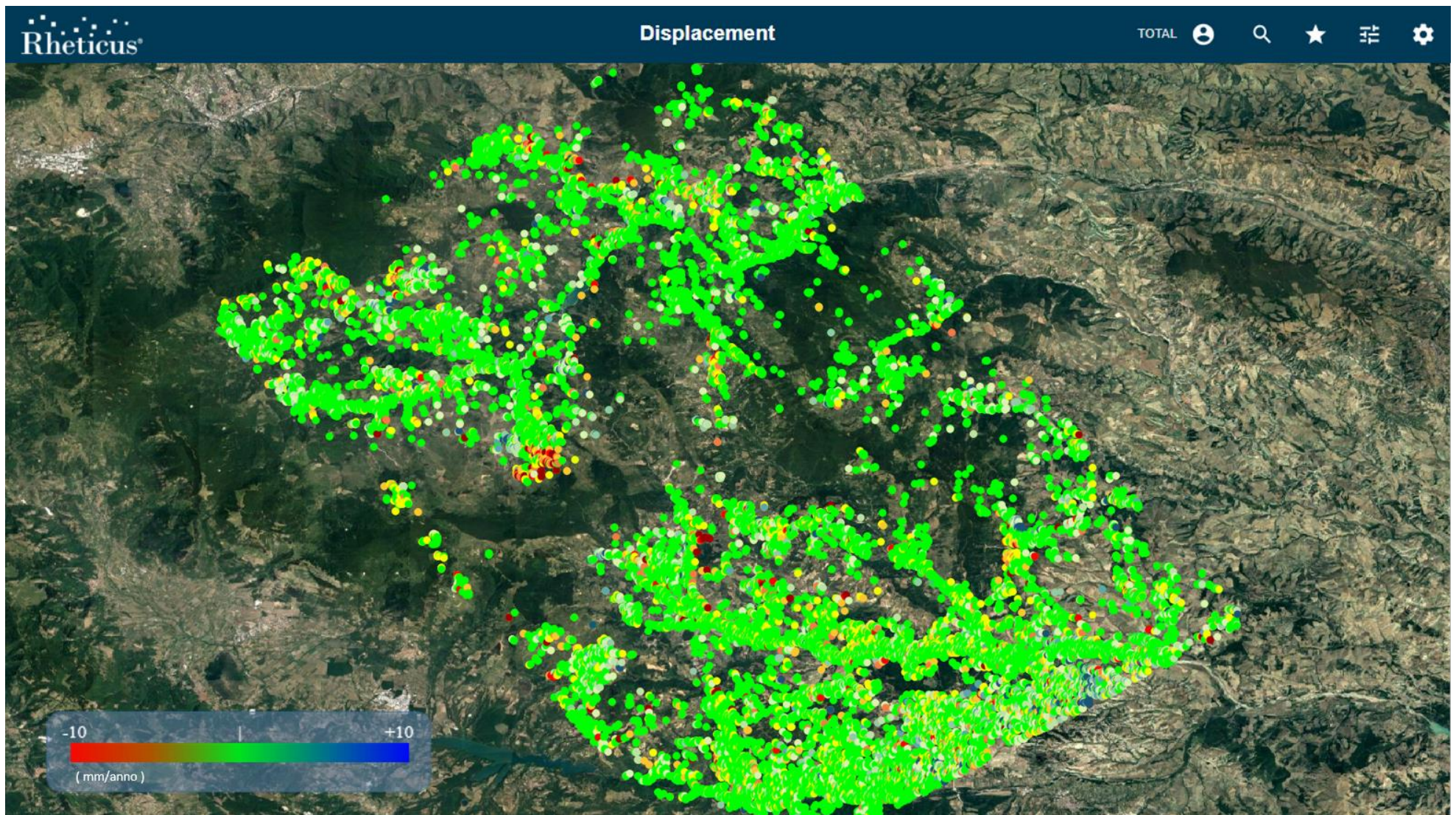
Figura 6: Mappa velocità media annua (mm/anno) in direzione Est(+) - Ovest(-) sul periodo esteso a Dicembre 2022 ottenuta dalla combinazione delle immagini Ascending e Descending acquisite dal satellite Sentinel-1.
