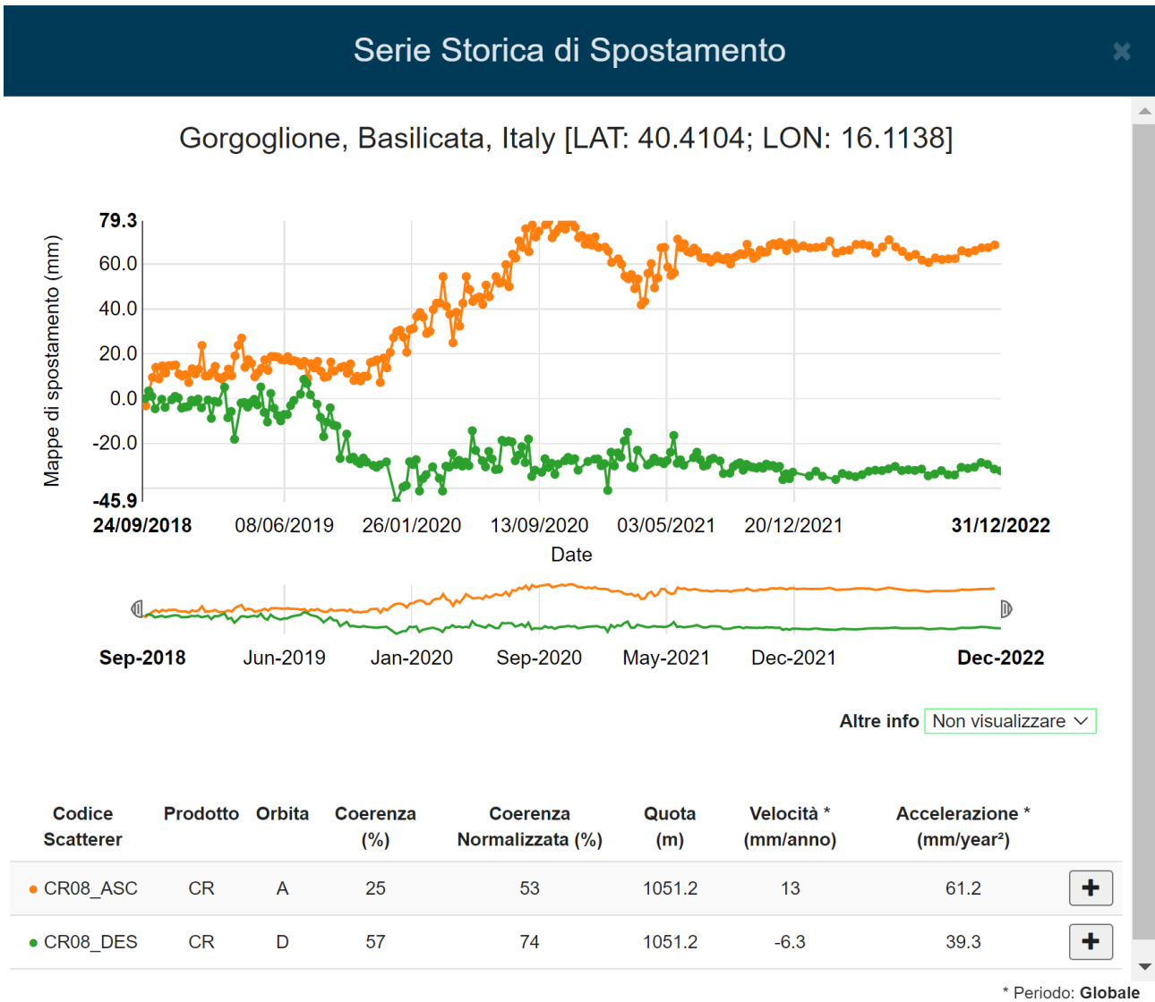
Figura 16: serie temporale di spostamento relativa al periodo settembre 2018 – Dicembre 2022 misurata in corrispondenza del Corner Reflector CR08. La serie temporale di spostamento in arancione è relativa all'orbita Ascending mentre quella verde rappresenta la serie temporale relativa all'orbita Descending.
