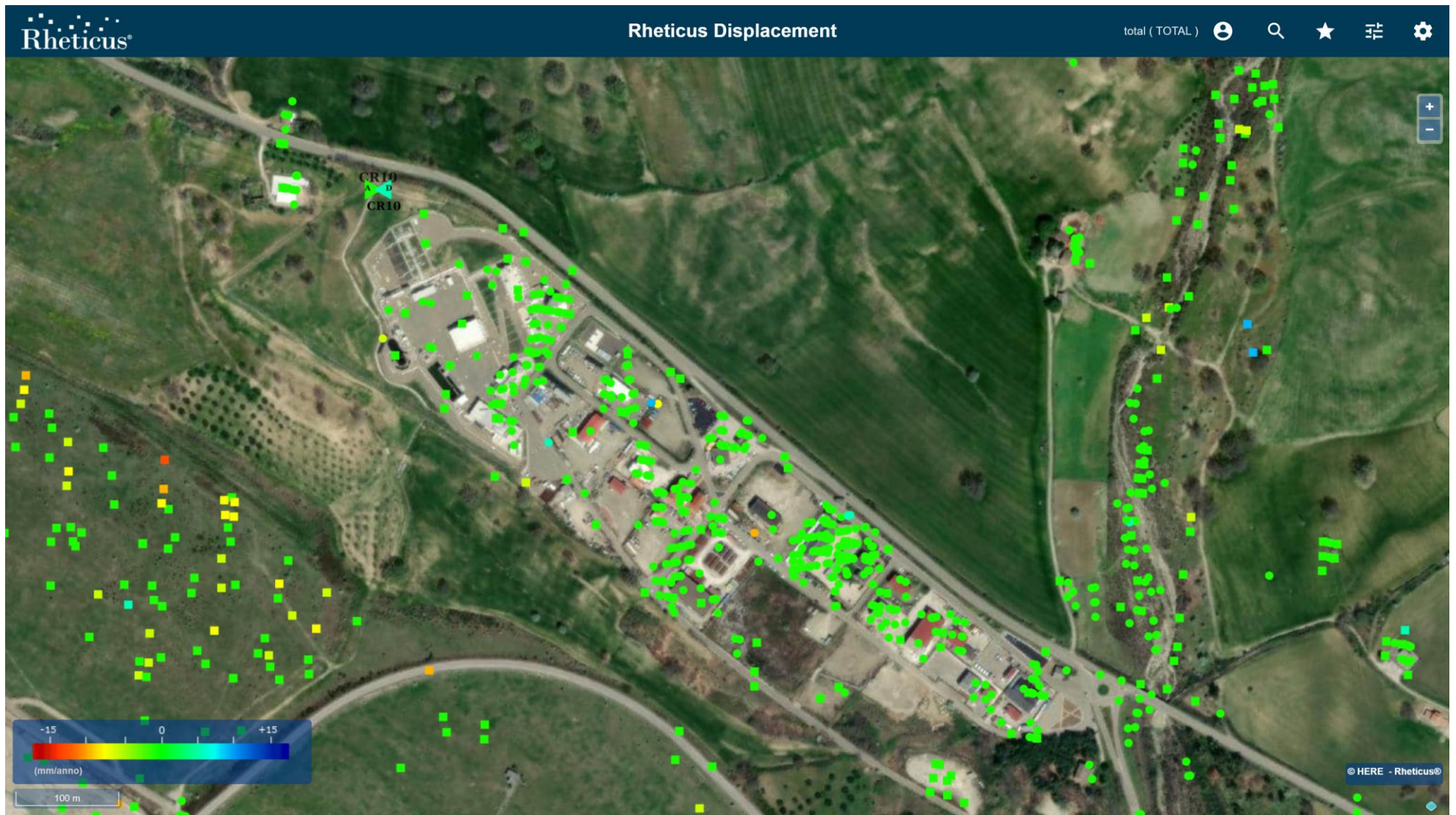
Figura 30: LPG Center caratterizzato da una buona copertura di PS e dai quali nel periodo esteso a Dicembre 2022, non si evincono variazioni significative di velocità media rispetto al precedente rapporto [RD13].
