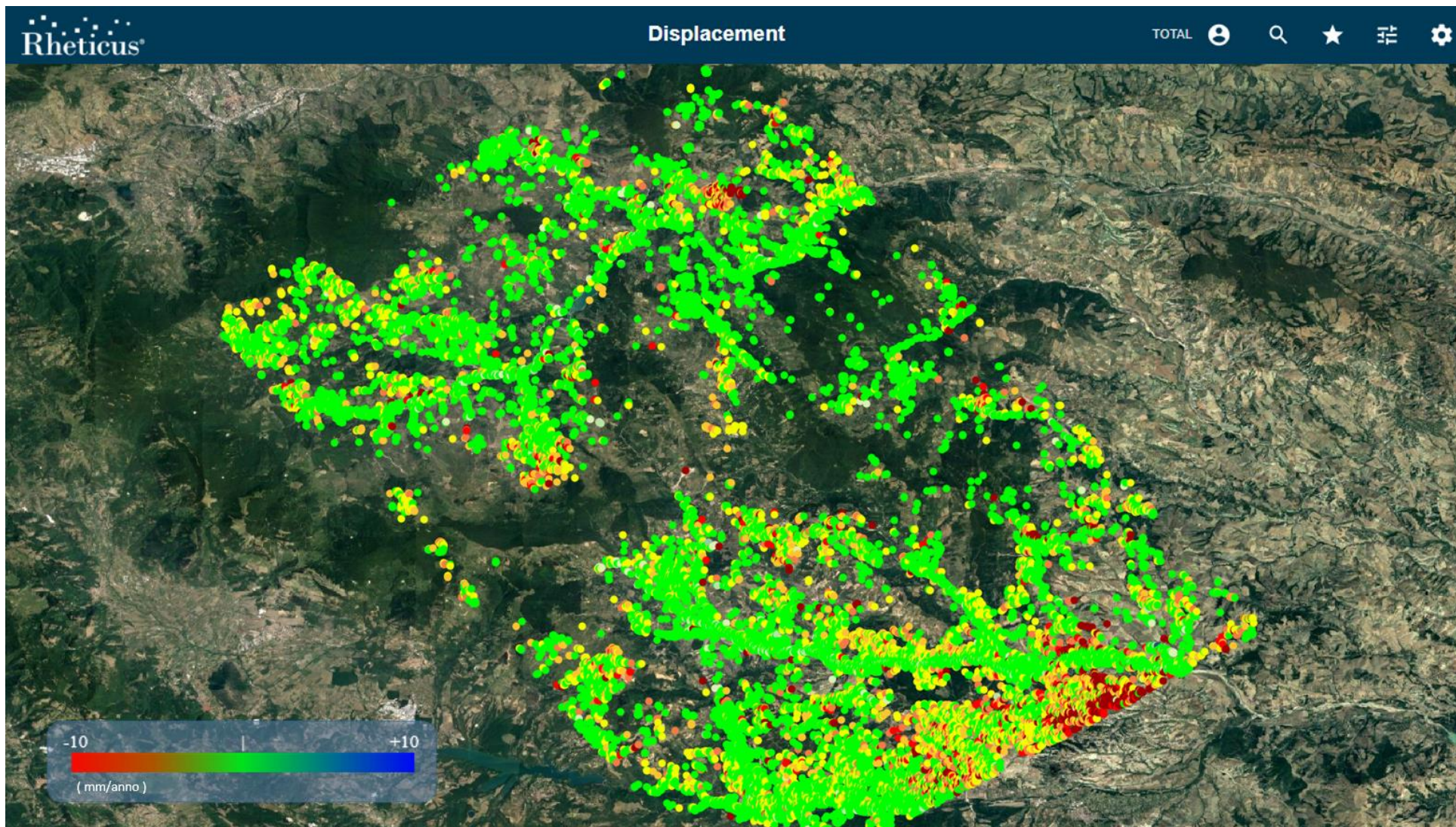
Figura 5: Mappa velocità media annua (mm/anno) lungo la direzione verticale sul periodo esteso a Dicembre 2022 ottenuta dalla combinazione delle immagini Ascending e Descending acquisite dal satellite Sentinel-1.
